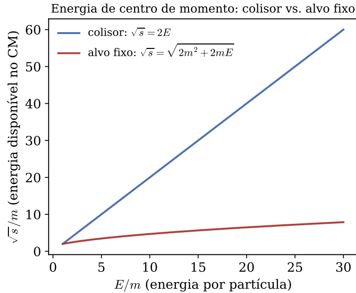
Figura 2.3. Energia disponível no referencial de centro de momento, \sqrt{s} , em função da energia E de cada partícula (mesma massa m nos dois casos). No colisor, \sqrt{s} = 2E cresce linearmente com E . No alvo fixo, \sqrt{s} = \sqrt{2m^2 + 2mE} cresce apenas com \sqrt{E} para E \gg m . A defasagem entre as duas curvas é exatamente a energia “desperdiçada” em manter o centro de momento em movimento no laboratório.
