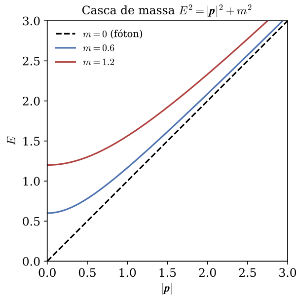
Figura 2.4. Casca de massa E^2 = |\mathbf{p}|^2 + m^2 no plano (|\mathbf{p}|, E) . Para m > 0 a curva é um ramo de hipérbole que nunca toca a reta E = |\mathbf{p}| ; por maior que seja o momento, E > |\mathbf{p}| sempre. Para m = 0 a casca degenera na própria reta E = |\mathbf{p}| — não há “folga” entre energia e momento para o fóton.
