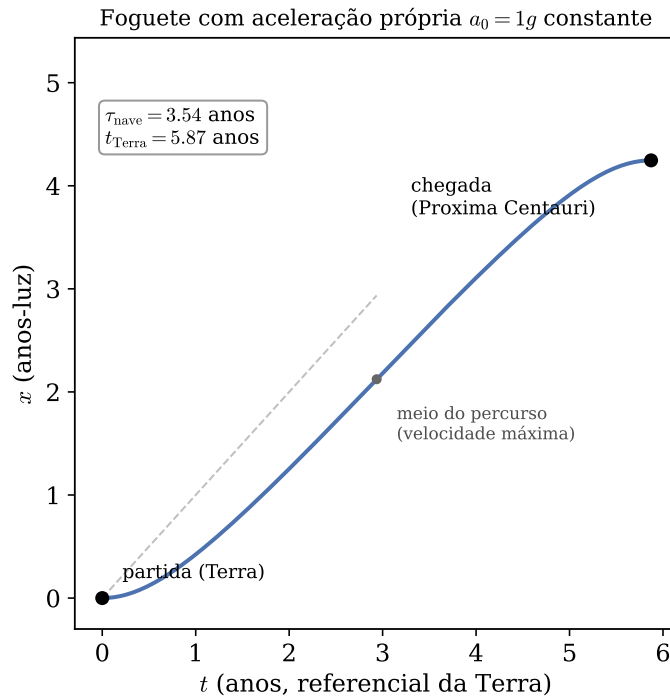
Figura 2.6. Trajetória no plano (t, x) do referencial da Terra para uma nave com aceleração própria constante a_0 = 1g , acelerando até o meio do percurso e desacelerando depois, para alcançar Proxima Centauri ( D = 4,25 anos-luz) em repouso. A reta tracejada é o cone de luz ( x = t ): a trajetória nunca a alcança.
