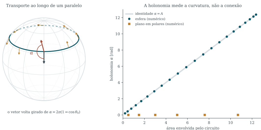
Figura 6.1. À esquerda, o vetor transportado ao longo de um paralelo da esfera: ele gira continuamente e não retorna à direção inicial. À direita, a holonomia medida contra a área envolvida pelo circuito. Os pontos da esfera caem sobre a reta \alpha = A — a curvatura de Gauss é 1 e a holonomia é a área. Os quadrados são o plano euclidiano em coordenadas polares: símbolos de Christoffel não nulos, holonomia nula para qualquer circuito.
