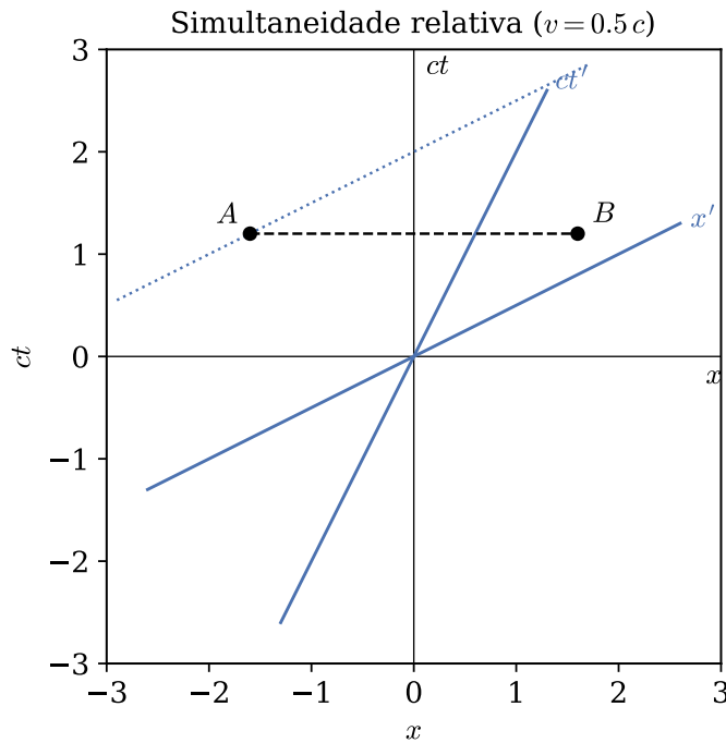
Figura 1.3. Diagrama de Minkowski: os eixos \bar{ct} e \bar{x} de \bar{S} aparecem inclinados em relação aos eixos de S pelo mesmo ângulo \arctan v . A reta tracejada liga dois eventos A e B simultâneos em S (mesma ct ); a reta pontilhada é a reta de simultaneidade de \bar{S} passando por A – ela não contém B .
