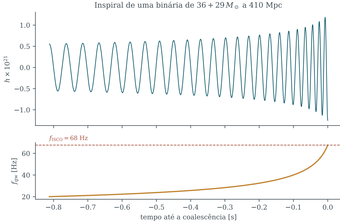
Figura 9.2. Acima, a forma de onda h(t) da binária de 36 + 29 M_{\odot} a 410 Mpc; abaixo, a frequência. Amplitude e frequência crescem juntas, e é daí que vem o nome chirp . A integração para em f_{\text{ISCO}} = 68 \text{ Hz} , onde a aproximação de órbita quase newtoniana deixa de valer e só a relatividade numérica descreve o que acontece.
