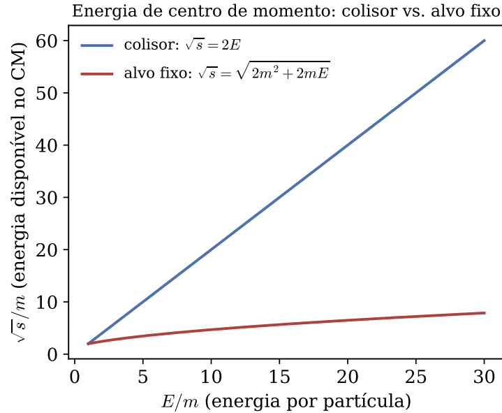
Figura 2.1. Energia disponível no referencial de centro de massa, \sqrt{s} , em função da energia E de cada partícula (mesma massa m nos dois casos). No colisor, \sqrt{s} = 2E cresce linearmente com E . No alvo fixo, \sqrt{s} = \sqrt{2m^2 + 2mE} cresce apenas com \sqrt{E} para E \gg m . A defasagem entre as duas curvas é exatamente a energia “desperdiçada” em manter o centro de massa em movimento no laboratório.
