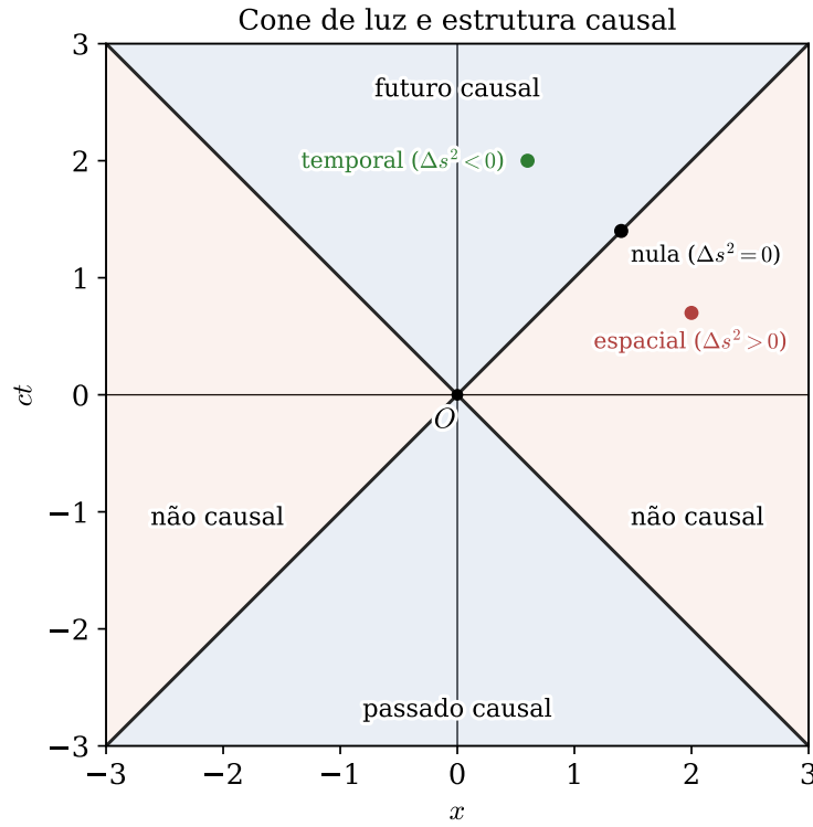
Figura 1.4. Cone de luz do evento O no plano (x, ct) . Eventos no futuro ou passado causal de O têm separação temporal; os eventos das duas cunhas laterais têm separação espacial e não podem ser causalmente ligados a O — daí o rótulo “não causal”. Os três pontos marcados retomam os Exemplos resolvidos desta seção.
