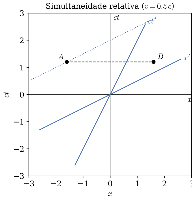
Figura 1.2. Diagrama de Minkowski: os eixos ct' e x' de S' aparecem inclinados em relação aos eixos de S pelo mesmo ângulo \arctan v . A reta tracejada liga dois eventos A e B simultâneos em S (mesma ct ); a reta pontilhada é a reta de simultaneidade de S' passando por A – ela não contém B .
