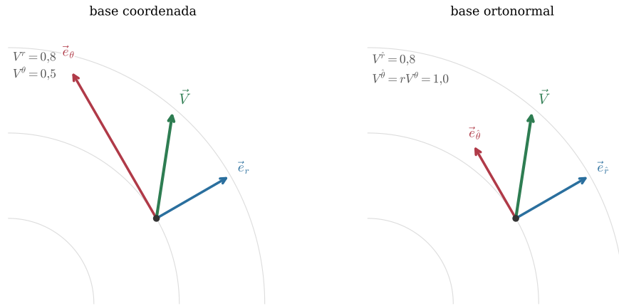
Figura 5.6. O mesmo vetor, no mesmo ponto, decomposto nas duas bases. À esquerda, a base coordenada, com \vec{e}_\theta de comprimento r ; à direita, a base ortonormal, com \vec{e}_{\hat{\theta}} de comprimento 1. As componentes diferem pelo fator r de (5.24) — e as unidades também, o que é o ponto.
