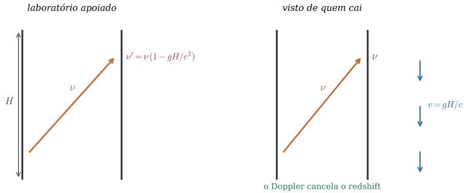
Figura 5.2. A mesma torre, vista do referencial que cai livremente. À esquerda, o laboratório apoiado: o fóton sobe e chega com frequência menor. À direita, visto de quem cai: no tempo de voo H/c o referencial adquiriu velocidade gH/c para baixo, e o Doppler correspondente cancela o redshift.
