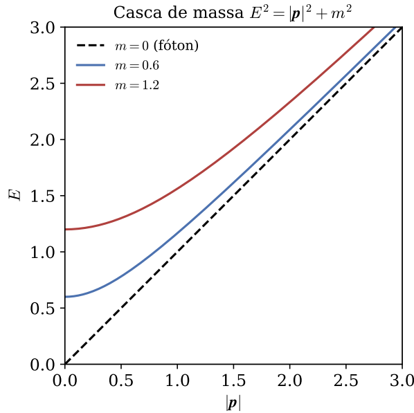
Figura 2.6. Casca de massa E^2 = |p|^2 + m^2 no plano (|p|, E) . Para m > 0 a curva é um ramo de hipérbole que nunca toca a reta E = |p| : por maior que seja o momento, E > |p| sempre. Para m = 0 a casca degenera na própria reta E = |p| — não há “folga” entre energia e momento para o fóton.
