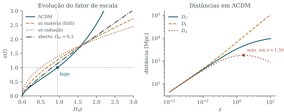
Figura 13.1. À esquerda, a(t) para quatro universos. Todos passam pela mesma origem, mas \Lambda CDM é o único que muda de concavidade: a curva desacelera enquanto a matéria domina e volta a acelerar depois. O universo aberto expande para sempre sem nunca acelerar. À direita, as três distâncias: D_L cresce sem limite, mas D_A tem um máximo em z \approx 1,59 — objetos mais distantes que isso aparecem maiores no céu.
