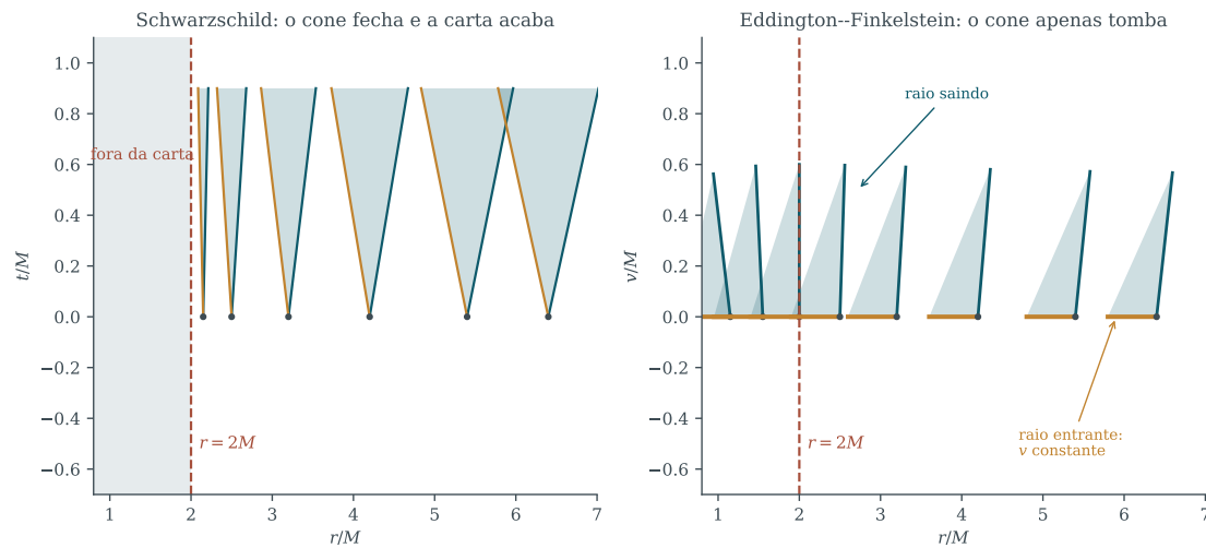
Figura 12.1. A mesma geometria em duas cartas. À esquerda, Schwarzschild: os cones se fecham ao se aproximarem de r = 2M e a região sombreada simplesmente não é coberta pelas coordenadas. À direita, Eddington-Finkelstein: os cones nunca se fecham, apenas tombam progressivamente; em r = 2M o raio que “sai” fica vertical, e para dentro os dois raios apontam para r decrescente.
