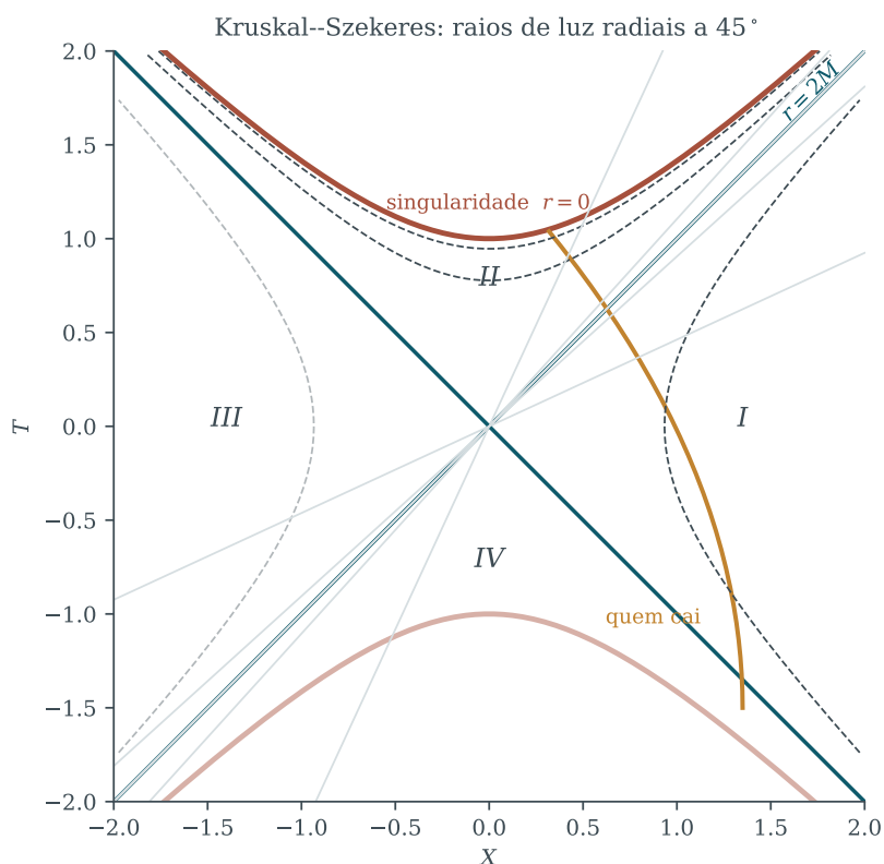
Figura 12.2. Diagrama de Kruskal-Szekeres, onde raios de luz radiais são retas a 45^\circ . As hipérboles tracejadas são r constante e as retas claras pela origem são t constante — note que todo o horizonte, para -\infty < t < \infty , colapsa nas duas diagonais. A linha de mundo em amarelo cruza o horizonte sem nada de particular e termina na singularidade, que é uma hipérbole horizontal : um instante no futuro, não um lugar no espaço.
