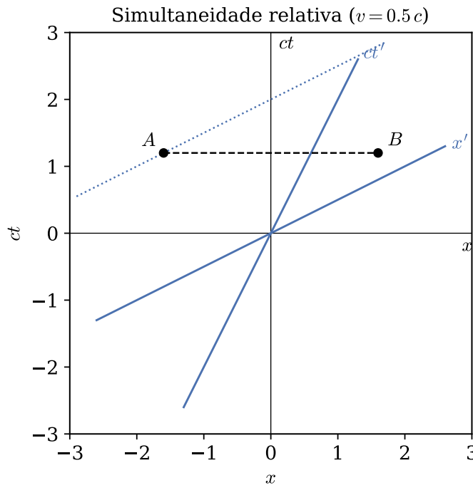
Figura 2.1. Diagrama de Minkowski: os eixos ct' e x' de S' aparecem inclinados em relação aos eixos de S pelo mesmo ângulo \arctan v . A reta tracejada liga dois eventos A e B simultâneos em S (mesma ct ); a reta pontilhada é a reta de simultaneidade de S' passando por A – ela não contém B .
