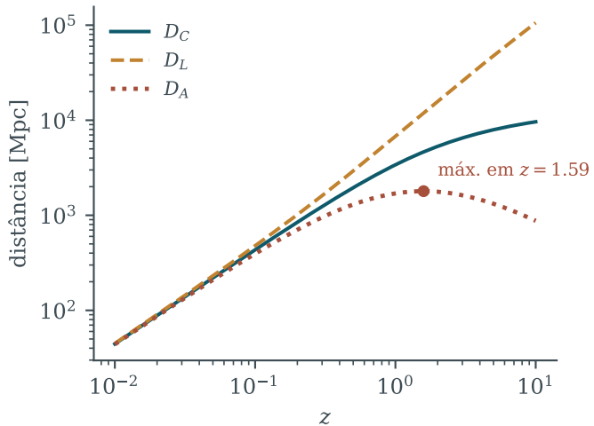
Distâncias em \Lambda CDM
