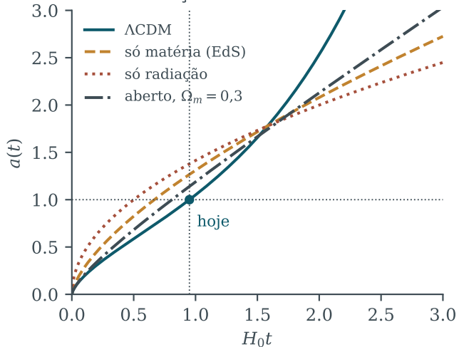
Evolução do fator de escala
