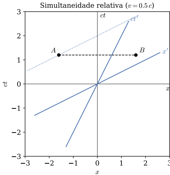
Figura 1.3. Diagrama de Minkowski: os eixos ct' e x' de \bar{S} aparecem inclinados em relação aos eixos de S pelo mesmo ângulo \arctan v . A reta tracejada liga dois eventos A e B simultâneos em S (mesma ct ); a reta pontilhada é a reta de simultaneidade de \bar{S} passando por A – ela não contém B .
