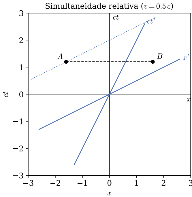
Figura 1.3. Diagrama de Minkowski: os eixos \bar{ct} e \bar{x} de \bar{S} aparecem inclinados em relação aos eixos de S pelo mesmo ângulo \arctan v . A reta tracejada liga dois eventos A e B simultâneos em S (mesma ct ); a reta pontilhada é a reta de simultaneidade de \bar{S} passando por A – ela não contém B .
