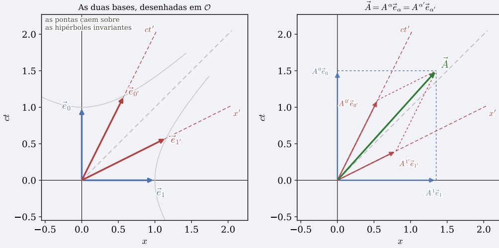
Figura 2.3. As duas bases e o mesmo vetor, tudo desenhado no papel de \mathcal{O} , com v = 0,5 . À esquerda, \vec{e}_0 e \vec{e}_1 apontam ao longo dos eixos \vec{t} e \vec{x} e têm as pontas sobre as hipérboles invariantes — parecem mais longos que \vec{e}_0 e \vec{e}_1 numa folha euclidiana, mas são igualmente unitários em Minkowski. À direita, a regra do paralelogramo nas duas bases devolve o mesmo \vec{A} , que é todo o conteúdo de \vec{A} = A^\alpha \vec{e}_\alpha = A'^\alpha \vec{e}'_\alpha . Numericamente, para o \vec{A} de componentes (1,5; 1,35; 0; 0) em \mathcal{O} , isso dá A^0 = 0,953 e A^1 = 0,693 .
