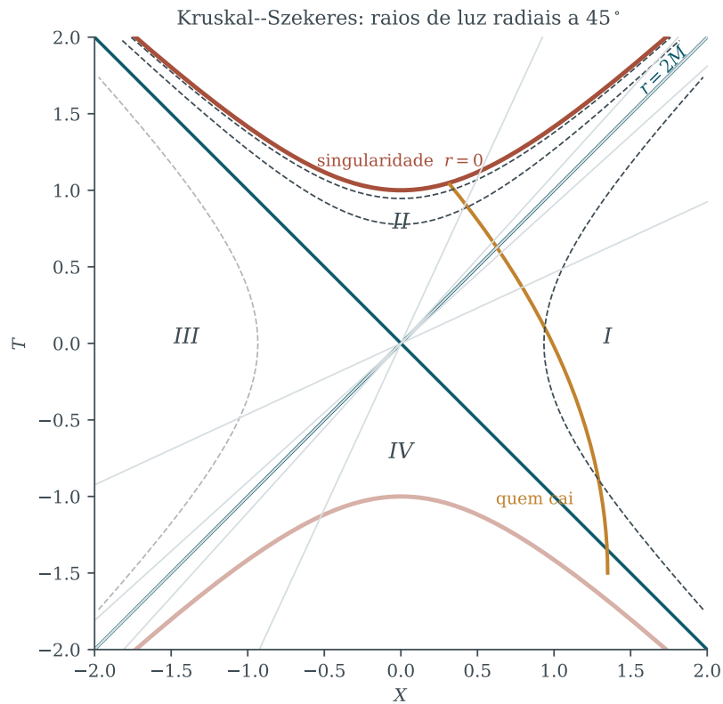
Figura 11.2. Diagrama de Kruskal-Szekeres, onde raios de luz radiais são retas a 45^\circ . As hipérboles tracejadas são r constante e as retas claras pela origem são t constante — note que todo o horizonte, para -\infty < t < \infty , colapsa nas duas diagonais. A linha de mundo em amarelo cruza o horizonte sem nada de particular e termina na singularidade, que é uma hipérbole horizontal : um instante no futuro, não um lugar no espaço.
