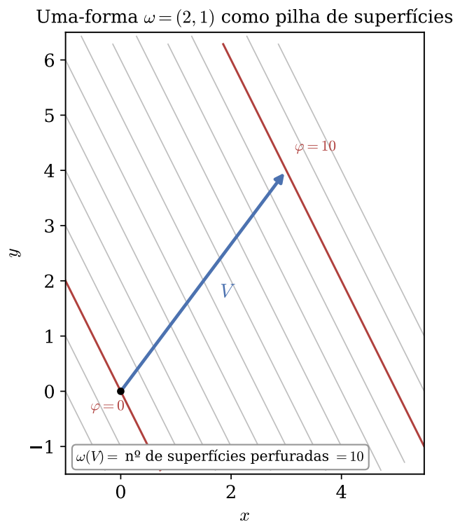
Figura 3.1. A 1-forma \tilde{\omega} , de componentes (2, 1) , representada como uma pilha de retas (superfícies de nível de \varphi = 2x + y , espaçadas de \Delta\varphi = 1 ). O vetor \vec{V} , de componentes (3, 4) , vai de \varphi = 0 a \varphi = 10 , perfurando exatamente 10 retas – por isso \tilde{\omega}(\vec{V}) = 10 . Esses são os mesmos \tilde{\omega} e \vec{V} do Exemplo 3.1.
