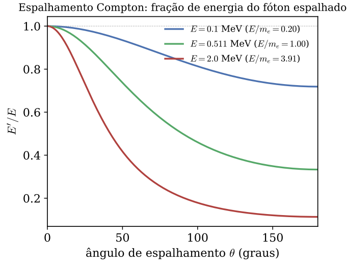
Figura 2.6. Fração de energia E'/E do fóton espalhado em função do ângulo \theta , para três energias incidentes. Quanto maior E/m_e , mais forte o espalhamento (curva mais baixa): no limite E \ll m_e (curva azul) o efeito quase desaparece e recupera-se o espalhamento Thomson clássico, E' \approx E .
