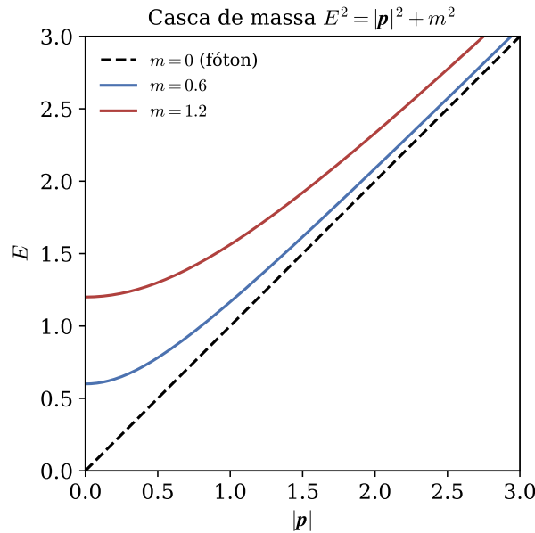
Figura 2.5. Casca de massa E^2 = |\mathbf{p}|^2 + m^2 no plano (|\mathbf{p}|, E) . Para m > 0 a curva é um ramo de hipérbole que nunca toca a reta E = |\mathbf{p}| : por maior que seja o momento, E > |\mathbf{p}| sempre. Para m = 0 a casca degenera na própria reta E = |\mathbf{p}| — não há “folga” entre energia e momento para o fóton.
