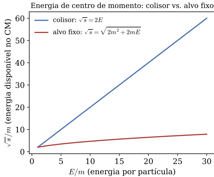
Figura 2.4. Energia disponível no referencial de centro de momento, \sqrt{s} , em função da energia E de cada partícula (mesma massa m nos dois casos). No colisor, \sqrt{s} = 2E cresce linearmente com E . No alvo fixo, \sqrt{s} = \sqrt{2m^2 + 2mE} cresce apenas com \sqrt{E} para E \gg m . A defasagem entre as duas curvas é exatamente a energia “desperdiçada” em manter o centro de momento em movimento no laboratório.
