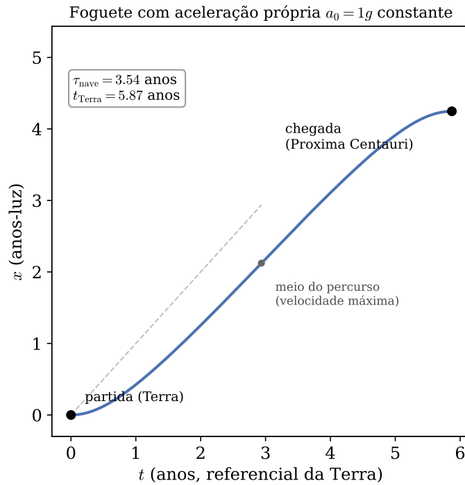
Figura 2.7. Trajetória no plano (t, x) do referencial da Terra para uma nave com aceleração própria constante a_0 = 1g , acelerando até o meio do percurso e desacelerando depois, para alcançar Proxima Centauri ( D = 4,25 anos-luz) em repouso. A reta tracejada é o cone de luz ( x = t ): a trajetória nunca a alcança.
