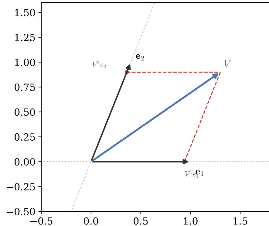
Componentes contravariantes V^i (paralelogramo)
