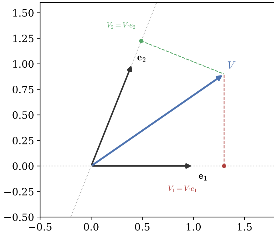
Componentes covariantes V_i (projeção perpendicular)
