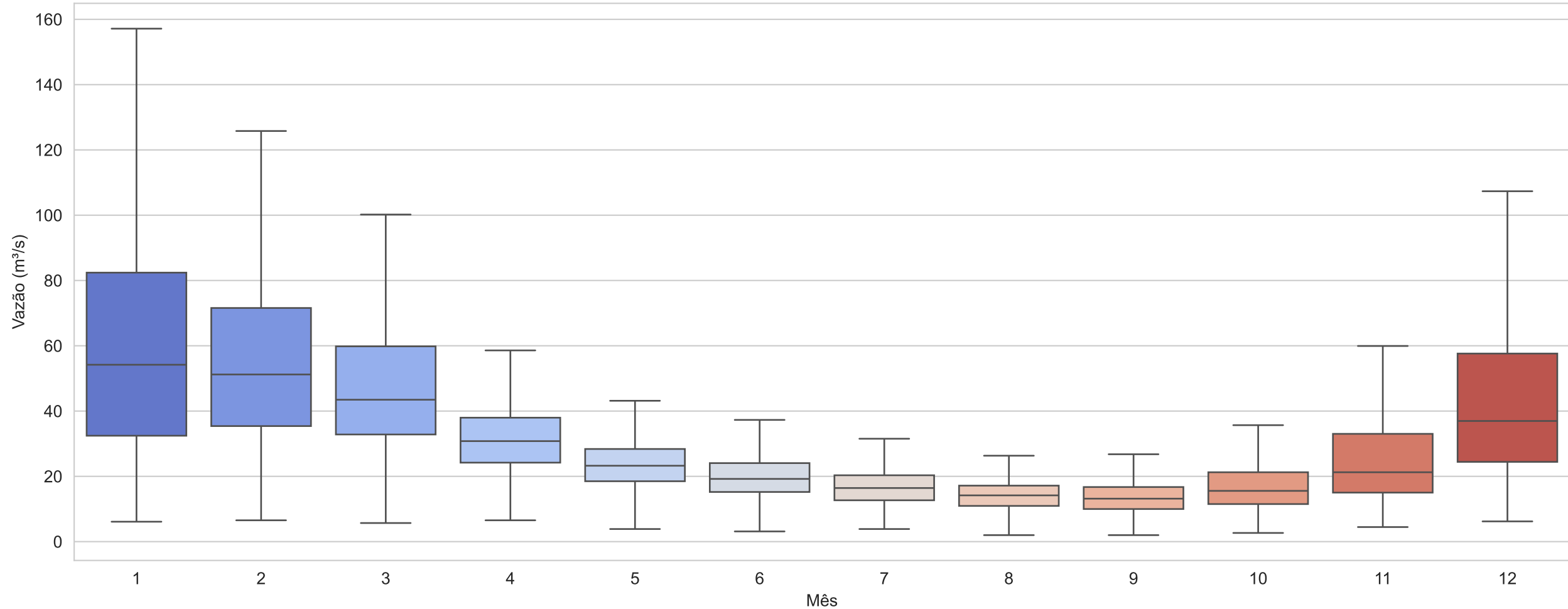
Boxplot Mensal da Vazão (sem outliers)
