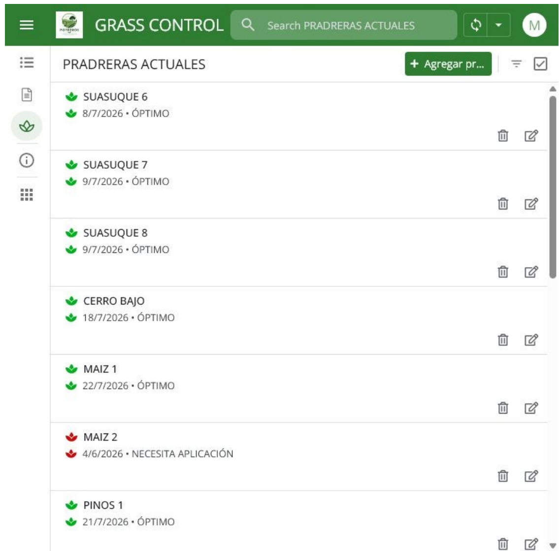
Figura 2. Vista principal PRADRERAS ACTUALES.
