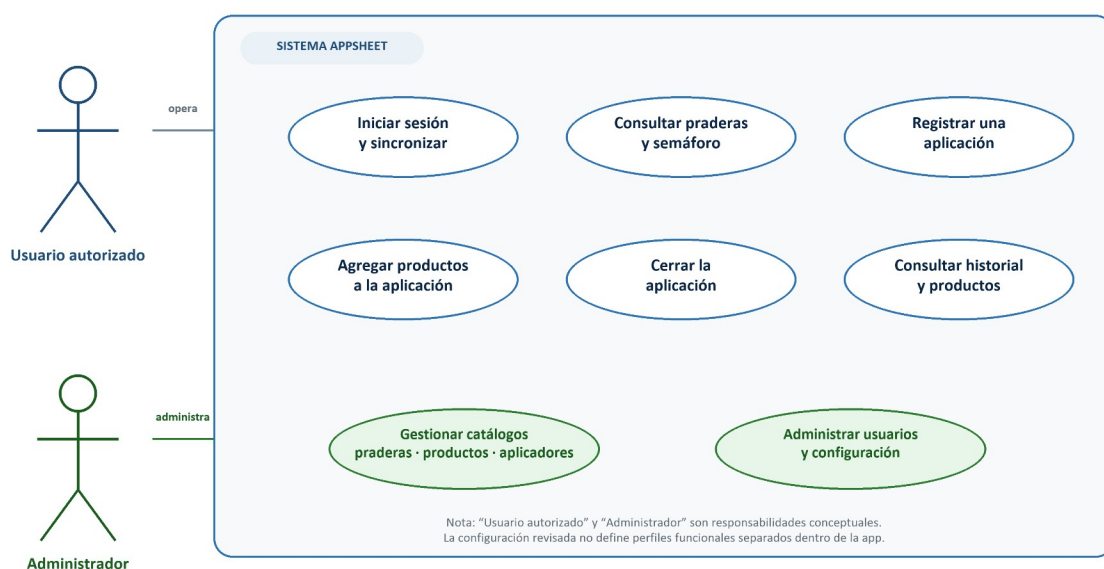
Figura 1. Casos de uso y responsabilidades operativas.
