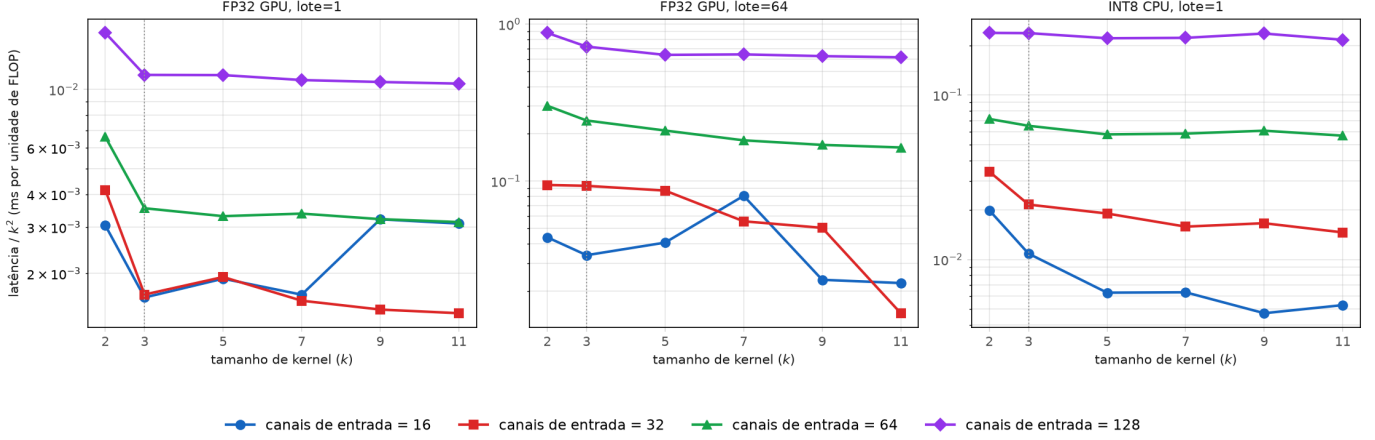
Figura 2. Latência por FLOP vs. tamanho de kernel (RTX 4060). O scaling sub-linear esperado de Winograd aparece de forma inconsistente entre regimes — ver texto para o teste estatístico e sua limitação no regime compute-bound ( batch =64, painel central).
