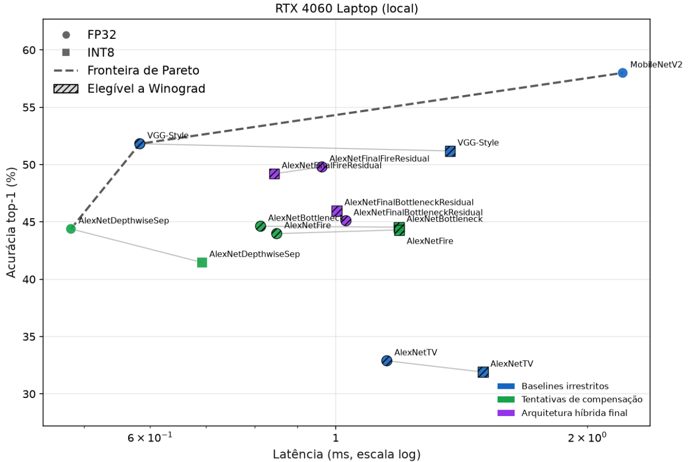
Figura 3. Fronteira de Pareto acurácia \times latência (FP32 e INT8, RTX 4060, batch=1 ). Cor indica o mesmo agrupamento da Figura 1 ( baselines irrestritos, restrição ingênua, tentativas de compensação, arquitetura híbrida final); forma indica precisão (círculo = FP32, quadrado = INT8); hachura indica elegibilidade arquitetural a Winograd (convolução 3 \times 3 de stride 1 densa presente) — não o traço medido de acionamento real (Eixo 3), mesma convenção da Figura 4. Nem todos os modelos aqui são elegíveis: MobileNetV2 (pointwise/depthwise) e AlexNetDepthwiseSep ficam sem hachura. Modelos com convolução 3 \times 3 densa ( bottleneck , Fire) atingem latência competitiva com trade-off de acurácia face ao baseline irrestrito; modelos depthwise não recebem aceleração Winograd apesar do kernel pequeno.
