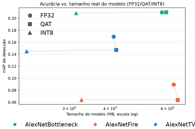
Figura 7. Detecção: acurácia (mAP) vs. tamanho real do modelo (tamanho real medido, que exclui os pesos do classificador pré-treinado nunca usados no forward pass de detecção), FP32, QAT e INT8, para os três backbones .
