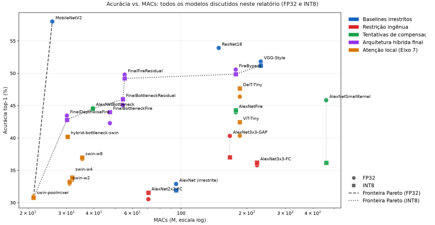
Figura 5. Acurácia vs. MACs (M, escala log) para 22 modelos — os 15 das Fases 1–4 e 9 mais os sete modelos de atenção local do Eixo 7 — do conjunto completo comparado por tamanho na Figura 4. MACs não muda entre FP32 e INT8 — mesma arquitetura, mesma contagem de multiplicação-acumulação — por isso os pontos FP32/INT8 de cada modelo compartilham a mesma posição no eixo X, unidos por uma linha vertical em vez da diagonal usada na Figura 4. Fronteira de Pareto tracejada (FP32) / pontilhada (INT8); um rótulo por modelo, posicionado sobre o ponto mais alto do par.
