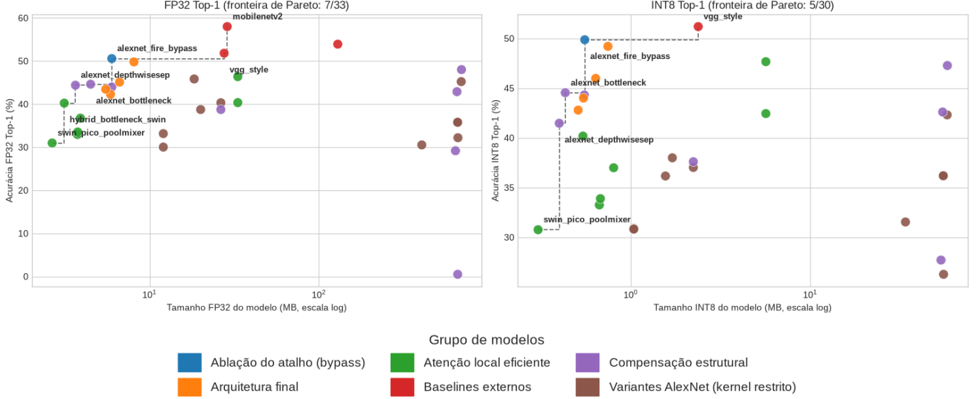
Figura 4. Acurácia top-1 vs. tamanho do checkpoint (MB, escala log) para os 33 modelos de classificação deste estudo (Fases 1–4, 8 e 9; o Eixo 6 mede mAP/mIoU, não top-1, e por isso não é comparável nesta mesma escala — omitida aqui). Dois painéis, FP32 (esquerda) e INT8 (direita), cada um com sua própria fronteira de Pareto tamanho-acurácia (linha tracejada; apenas os modelos na fronteira são rotulados, para legibilidade). Cor indica a fase de origem do modelo (mesma legenda em ambos os painéis). O painel INT8 tem 5 de 30 modelos na fronteira (contra 7 de 33 em FP32) e apenas 30 dos 33 modelos aparecem — MobileNetV2 e ResNet18 pré-treinados nunca passaram por QAT ( residual adds sem FloatFunctional , Seção III-A).
