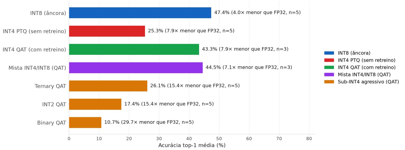
Figura 6. Acurácia top-1 média por método de compressão além de INT8, com taxa de compressão (tamanho do checkpoint FP32 dividido pelo tamanho do checkpoint comprimido) e número de modelos ( n ) entre parênteses. INT4 PTQ (sem retreino) colapsa para 25,3%; retreinar sob o mesmo INT4 (QAT) recupera para 43,3% — o retreino, não a largura de bits em si, é o que preserva a acurácia. Precisão mista INT4/INT8 (QAT) supera até o INT4 QAT uniforme com taxa de compressão comparável. Métodos sub-INT4 mais agressivos (ternary, int2, binary, todos QAT) degradam progressivamente.
