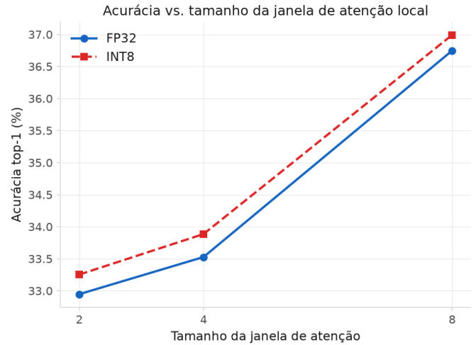
Figura 8. Acurácia top-1 (FP32 e INT8) vs. tamanho de janela de atenção local \in \{2, 4, 8\} — análogo, em atenção, da curva de restrição de kernel do Eixo 1.
