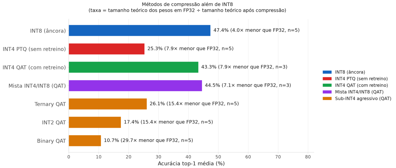
Figura 6. Acurácia top-1 média por método de compressão além de INT8, com taxa de compressão (tamanho teórico dos pesos em FP32 dividido pelo tamanho teórico após compressão) e número de modelos ( n ) entre parênteses. INT4 PTQ (sem retreino) colapsa para 25,3%; retreinar sob o mesmo INT4 (QAT) recupera para 43,3% — o retreino, não a largura de bits em si, é o que preserva a acurácia. As duas médias cobrem conjuntos de modelos diferentes ( n=5 vs. n=3 ); restrita aos 3 modelos com as duas medições, a recuperação vai de 27,7% para 43,3%. Precisão mista INT4/INT8 (QAT) supera até o INT4 QAT uniforme com taxa de compressão comparável. Métodos sub-INT4 mais agressivos (ternary, int2, binary, todos QAT) degradam progressivamente.
