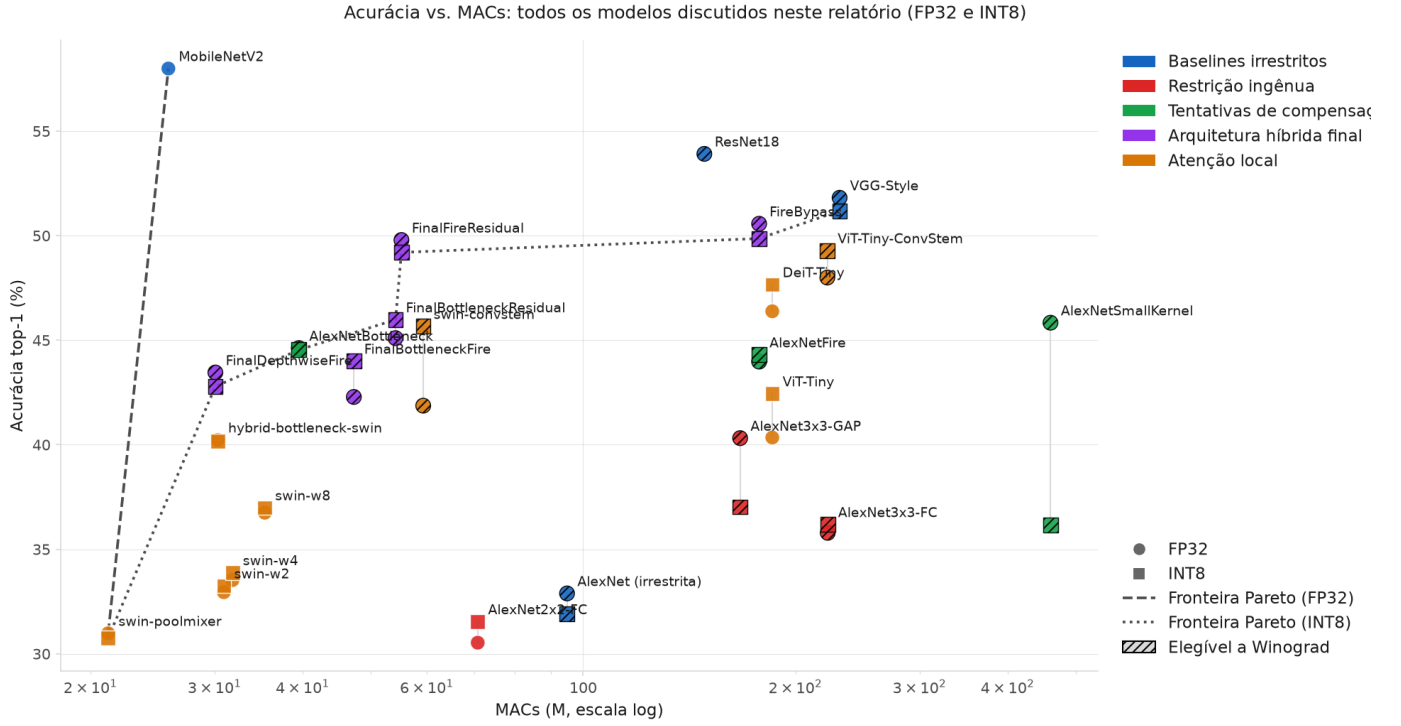
Figura 5. Acurácia vs. MACs (M, escala log) para 24 modelos — os 15 das Fases 1–4 e 9 mais os nove modelos de atenção local do Eixo 7, incluindo o contrafactual vit_tiny_convstem/swin_pico_convstem — do conjunto completo comparado por tamanho na Figura 4. MACs não muda entre FP32 e INT8 — mesma arquitetura, mesma contagem de multiplicação-acumulação — por isso os pontos FP32/INT8 de cada modelo compartilham a mesma posição no eixo X, unidos por uma linha vertical em vez da diagonal usada na Figura 4. Fronteira de Pareto tracejada (FP32) / pontilhada (INT8); um rótulo por modelo, posicionado sobre o ponto mais alto do par. Hachura indica elegibilidade arquitetural a Winograd (convolução 3 \times 3 de stride 1 densa presente), não o traço medido de acionamento, mesma convenção da Figura 4.
