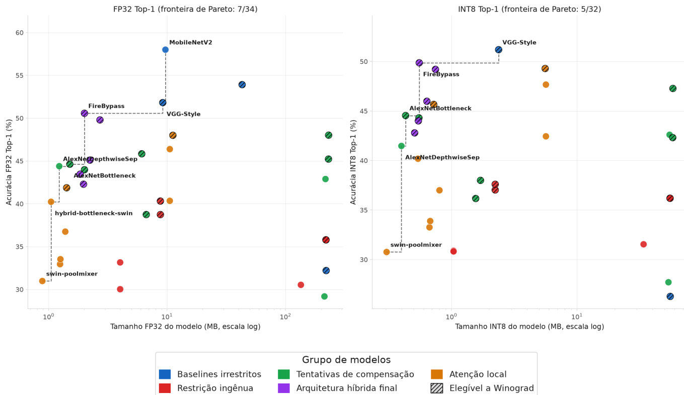
Figura 4. Acurácia top-1 vs. tamanho do modelo (pesos, MB, escala log) para os 34 modelos de classificação deste estudo (Fases 1–4, 8 e 9, incluindo o contrafactual vit_tiny_convstem/swin_pico_convstem ; omitidos: o Eixo 6, que mede mAP/mIoU, não top-1, e por isso não é comparável nesta mesma escala, e AlexNetSE, cujo treino malsucedido ( \sim 0.5\% top-1, Tabela XI) não é um ponto real de eficiência). Três dos 34 pontos ( alexnet_2x2 , alexnet_3x3 , alexnet_gap ) são reexecuções curtas superadas de arquiteturas já presentes na figura ( AlexNet2x2-GAP , AlexNet3x3-FC , AlexNet3x3-GAP ): mesma arquitetura e mesmo tamanho, acurácia menor ou igual ( alexnet_3x3 repete o mesmo resultado FP32 de AlexNet3x3-FC ); nenhuma entra na fronteira. Dois painéis, FP32 (esquerda) e INT8 (direita), cada um com sua própria fronteira de Pareto tamanho-acurácia (linha tracejada; apenas os modelos na fronteira são rotulados, para legibilidade). Cor indica a fase de origem do modelo (mesma legenda em ambos os painéis); hachura indica elegibilidade arquitetural a Winograd (convolução 3 \times 3 de stride 1 densa presente) — não o traço medido de acionamento real (Eixo 3/7, disponível só para um subconjunto dos modelos aqui). O painel INT8 tem 5 de 32 modelos na fronteira (contra 7 de 34 em FP32) e apenas 32 dos 34 modelos aparecem — MobileNetV2 e ResNet18 pré-treinados nunca passaram por QAT ( residual adds sem operador de soma dedicado à quantização, Seção III-A).
