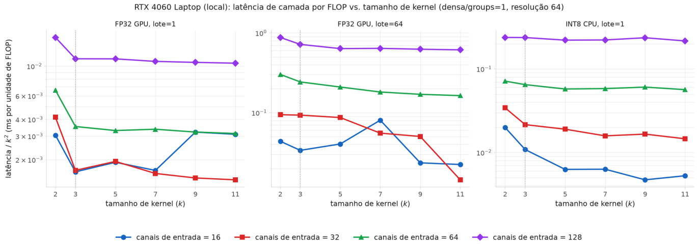
Figura 2. Latência por FLOP vs. tamanho de kernel (RTX 4060). O scaling sub-linear esperado de Winograd aparece de forma inconsistente entre regimes — ver texto para o teste estatístico e sua limitação no regime compute-bound ( batch =64, painel central).
