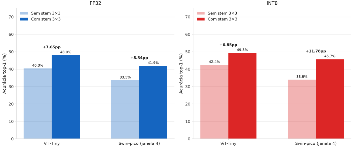
Figura 9. Ganho de acurácia top-1 (FP32 e INT8) ao acrescentar um stem 3×3 de stride 1 elegível a Winograd a vit_tiny e swin_pico (janela 4). O ganho não é grátis: a camada acrescenta MACs (+86% no swin_pico , +20% no vit_tiny ) e os orçamentos de treino diferem entre os pares — ver texto.
