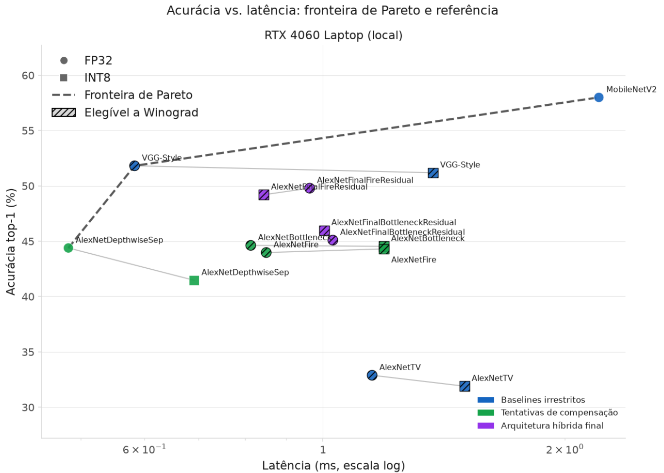
Figura 3. Fronteira de Pareto acurácia \times latência (FP32 e INT8, RTX 4060, batch=1 ). Cor indica o mesmo agrupamento da Figura 1 ( baselines irrestritos, restrição ingênua, tentativas de compensação, arquitetura híbrida final); forma indica precisão (círculo = FP32, quadrado = INT8); hachura indica elegibilidade arquitetural a Winograd (convolução 3 \times 3 de stride 1 densa presente) — não o traço medido de acionamento real (Eixo 3), mesma convenção da Figura 4. Nem todos os modelos aqui são elegíveis: MobileNetV2 (pointwise/depthwise) e AlexNetDepthwiseSep ficam sem hachura. Modelos com convolução 3 \times 3 densa ( bottleneck , Fire ) atingem latência competitiva com trade-off de acurácia face ao baseline irrestrito; modelos depthwise não recebem aceleração Winograd apesar do kernel pequeno.
