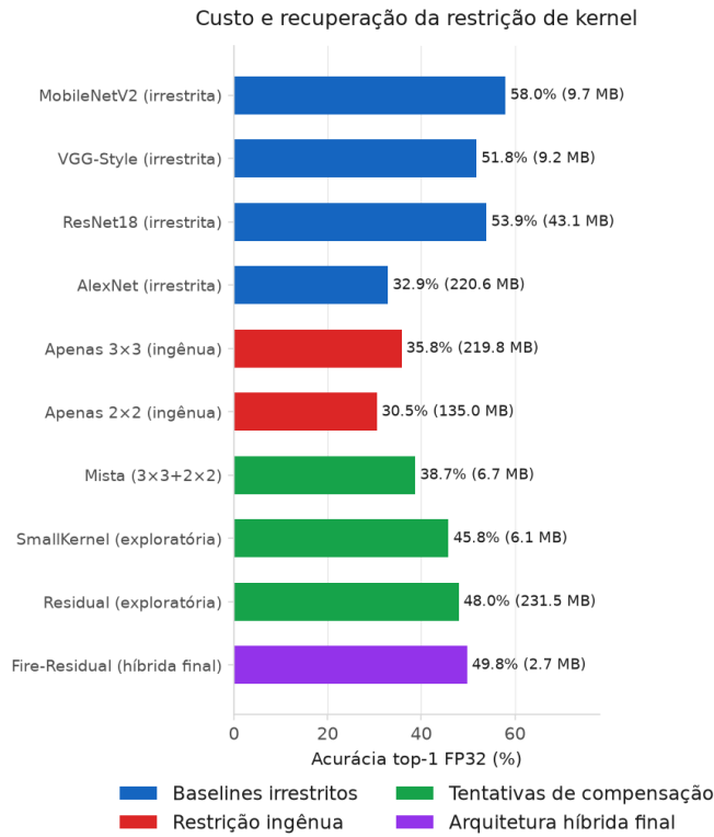
Figura 1. Acurácia FP32 (top-1) por arquitetura, contrastando baselines externos de kernel irrestrito (MobileNetV2, ResNet18, VGG-Style), restrição ingênuo (AlexNet 3×3 e 2×2), tentativas exploratórias de compensação (Mixed, Residual puro — não detalhadas individualmente neste relatório; SmallKernel é retomado com números no Eixo 5) e a arquitetura híbrida final (Fire-Residual).
