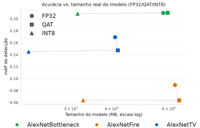
Figura 7. Detecção: acurácia (mAP) vs. tamanho real do modelo (tamanho real medido, que exclui os pesos do classificador pré-treinado nunca usados no forward pass de detecção), FP32, QAT e INT8, para os três backbones .
