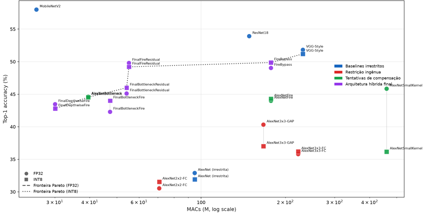
Figura 5. Acúrcia vs. MACs (M, escala log) para um subconjunto de 15 modelos (Fases 1–4 e 9) do conjunto completo de 33 modelos comparado por tamanho na Figura 4; os sete modelos de atenção do Eixo 7 têm MACs tabulados separadamente (Tabela IX), não neste gráfico. MACs não muda entre FP32 e INT8 — mesma arquitetura, mesma contagem de multiplicação-acumulação — por isso os pontos FP32/INT8 de cada modelo compartilham a mesma posição no eixo X, unidos por uma linha vertical em vez da diagonal usada na Figura 4. Fronteira de Pareto tracejada (FP32) / pontilhada (INT8); apenas os modelos na fronteira são rotulados.
