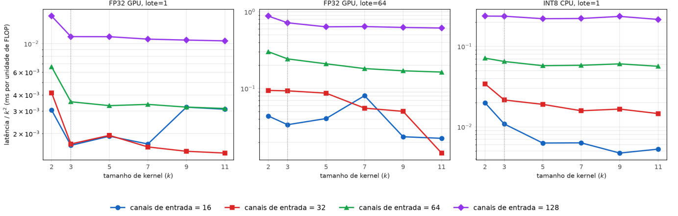
RTX 4060 Laptop (local): latência de camada por FLOP vs. tamanho de kernel (densa/groups=1, resolução 64)
