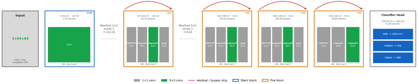
Figura 12. AlexNetFinalFireResidual: stem 3 \times 3\ stride\text{-}2 seguido de módulos Fire com atalho residual em cada estágio.
