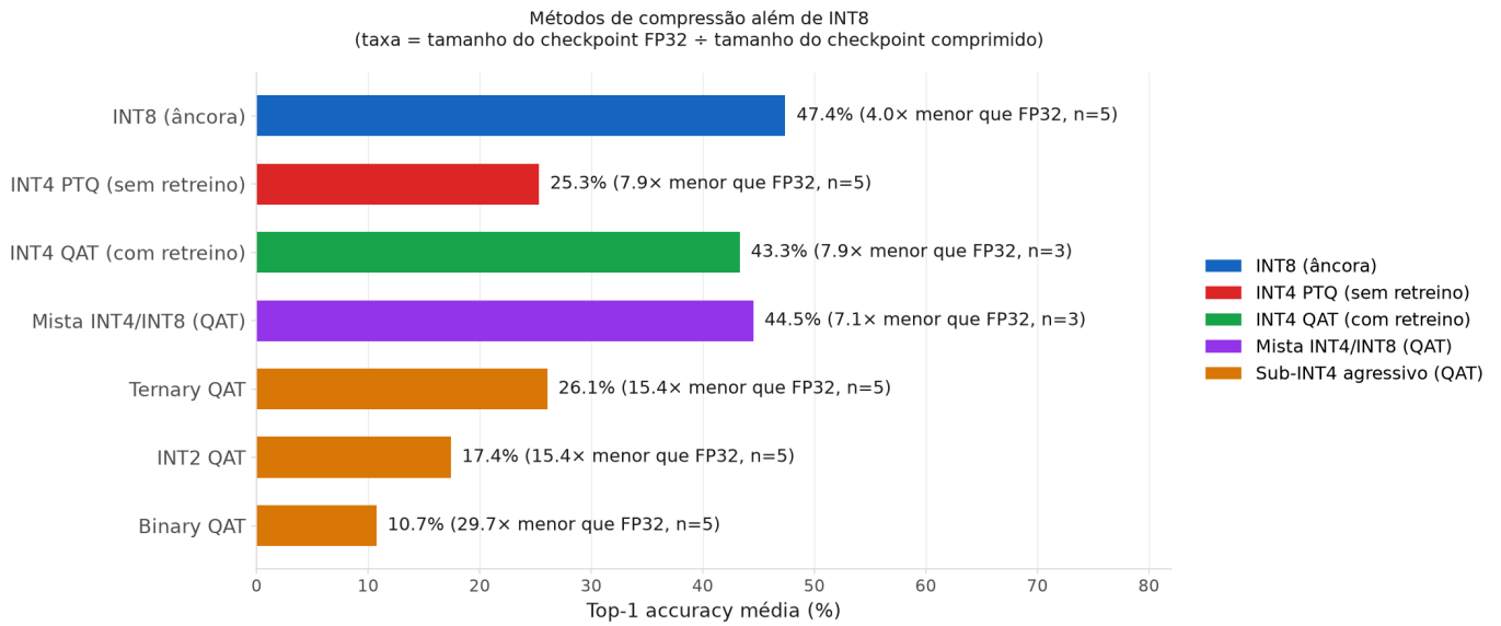
Figura 6. Acurácia top-1 média por método de compressão além de INT8, com taxa de compressão (tamanho do checkpoint FP32 dividido pelo tamanho do checkpoint comprimido) e número de modelos ( n ) entre parênteses. INT4 PTQ (sem retreino) colapsa para 25,3%; retreinar sob o mesmo INT4 (QAT) recupera para 43,3% — o retreino, não a largura de bits em si, é o que preserva a acurácia. Precisão mista INT4/INT8 (QAT) supera até o INT4 QAT uniforme com taxa de compressão comparável. Métodos sub-INT4 mais agressivos (ternary, int2, binary, todos QAT) degradam progressivamente.
