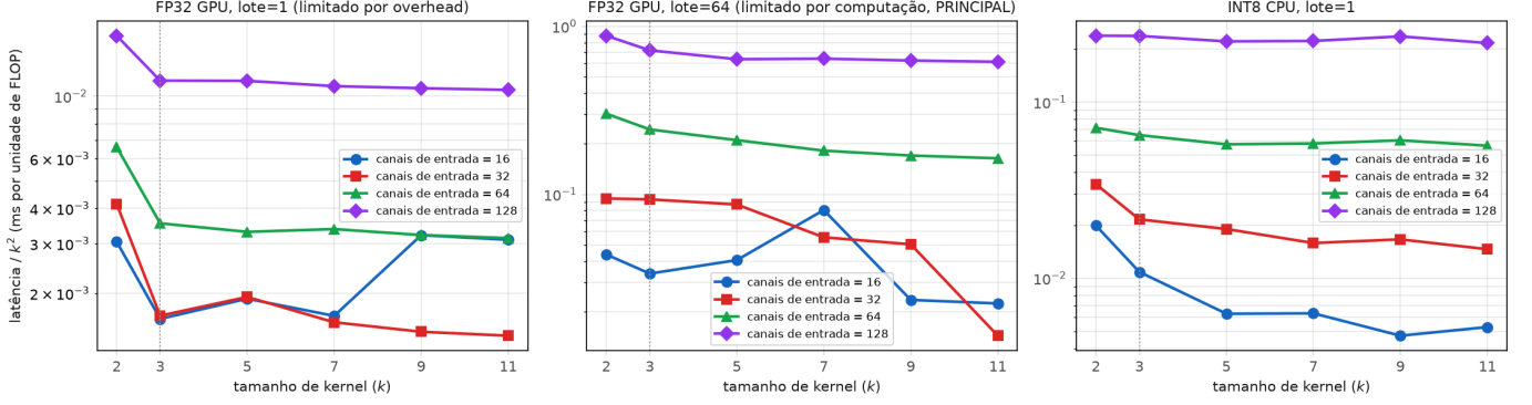
Figura 2. Latência por FLOP vs. tamanho de kernel (RTX 4060). O scaling sub-linear esperado de Winograd aparece de forma inconsistente entre regimes — ver texto para o teste estatístico e sua limitação no regime compute-bound ( \text{batch}=64 , painel central).
