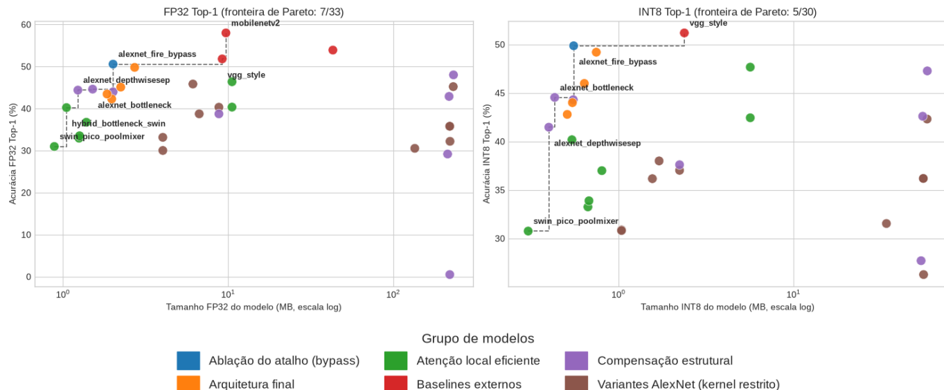
Figura 4. Acurácia top-1 vs. tamanho do modelo (pesos, MB, escala log) para os 33 modelos de classificação deste estudo (Fases 1–4, 8 e 9; o Eixo 6 mede mAP/mIoU, não top-1, e por isso não é comparável nesta mesma escala — omitida aqui). Dois painéis, FP32 (esquerda) e INT8 (direita), cada um com sua própria fronteira de Pareto tamanho-acurácia (linha tracejada; apenas os modelos na fronteira são rotulados, para legibilidade). Cor indica a fase de origem do modelo (mesma legenda em ambos os painéis). O painel INT8 tem 5 de 30 modelos na fronteira (contra 7 de 33 em FP32) e apenas 30 dos 33 modelos aparecem — MobileNetV2 e ResNet18 pré-treinados nunca passaram por QAT ( residual adds sem FloatFunctional , Seção III-A).
