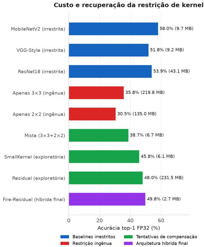
Figura 1. Acurácia FP32 (top-1) por arquitetura, contrastando baselines externos de kernel irrestrito (MobileNetV2, ResNet18, VGG-Style), restrição ingênua (AlexNet 3×3 e 2×2), tentativas exploratórias de compensação (Mixed, Residual puro — não detalhadas individualmente neste relatório; SmallKernel é retomado com números no Eixo 5) e a arquitetura híbrida final (Fire-Residual).
