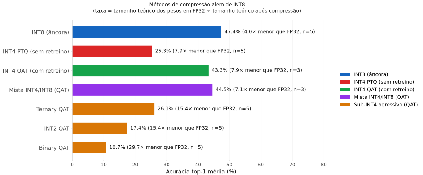
Figura 6. Acúrcia top-1 média por método de compressão além de INT8, com taxa de compressão (tamanho teórico dos pesos em FP32 dividido pelo tamanho teórico após compressão) e número de modelos ( n ) entre parênteses. INT4 PTQ (sem retreino) colapsa para 25,3%; retreinar sob o mesmo INT4 (QAT) recupera para 43,3% — o retreino, não a largura de bits em si, é o que preserva a acúrcia. Precisão mista INT4/INT8 (QAT) supera até o INT4 QAT uniforme com taxa de compressão comparável. Métodos sub-INT4 mais agressivos (ternary, int2, binary, todos QAT) degradam progressivamente.
