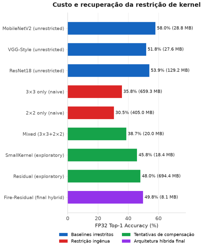
Figura 1. Acurácia FP32 (top-1) por arquitetura, contrastando baselines externos de kernel irrestrito (MobileNetV2, ResNet18, VGG-Style), restrição ingênua (AlexNet 3 \times 3 e 2 \times 2 ), tentativas exploratórias de compensação (Mixed, Residual puro — não detalhadas individualmente neste relatório; SmallKernel é retomado com números na Contribuição 5) e a arquitetura híbrida final (Fire-Residual).
