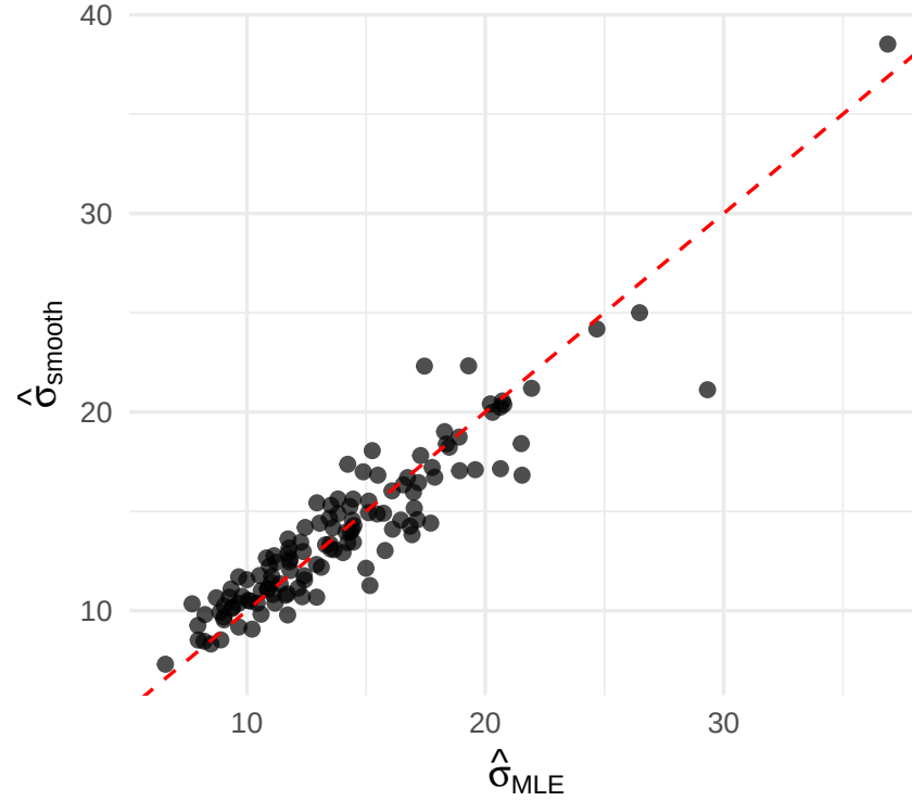
\sigma (scale)
