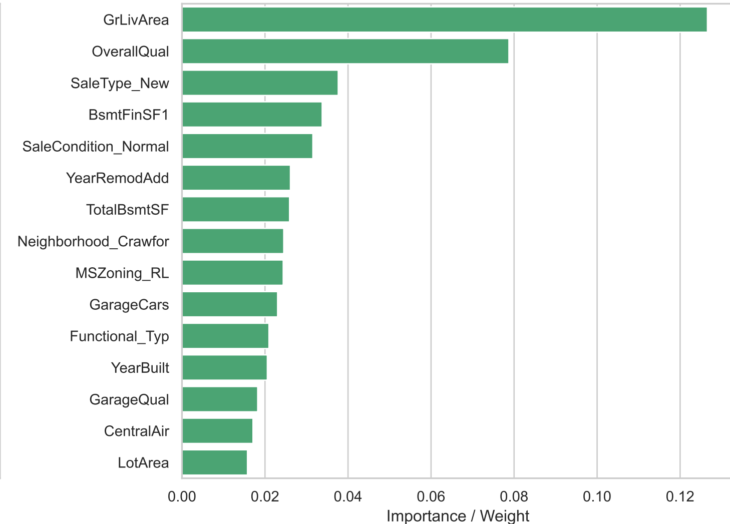
LassoCV: Top 15 Features
