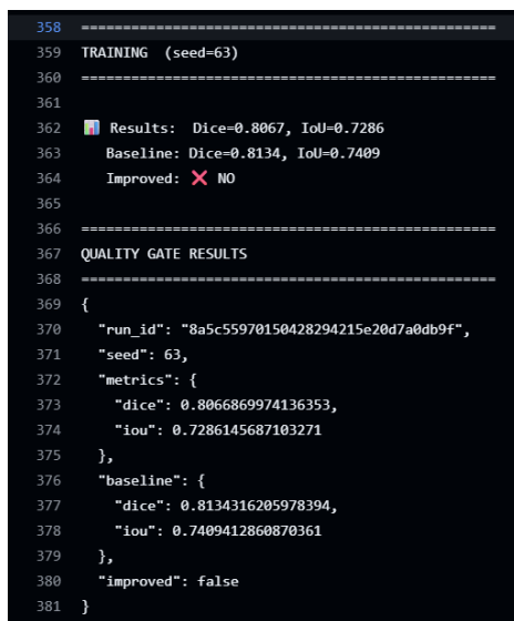
Rys. 15 Wynik bramki jakości — model nie spełnił kryteriów, więc nie został wdrożony
