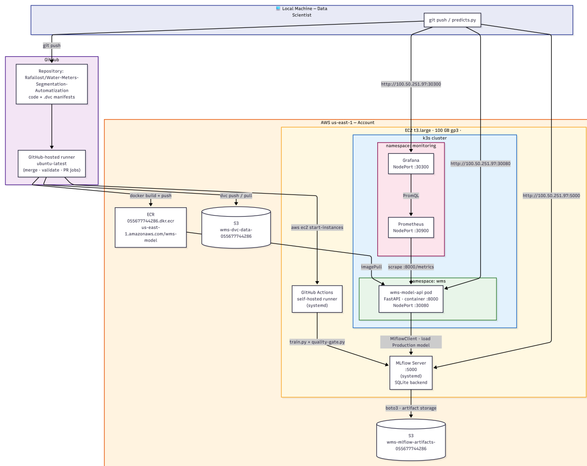
Rys. 15 Diagram wdrożenia systemu — konkretne zasoby AWS, adresy i porty.
