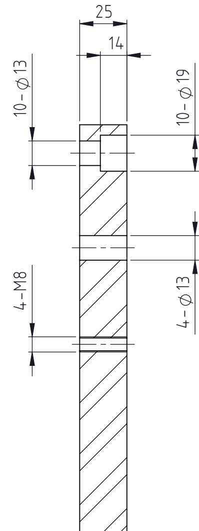
SECTION A-A SCALE 1 : 2
