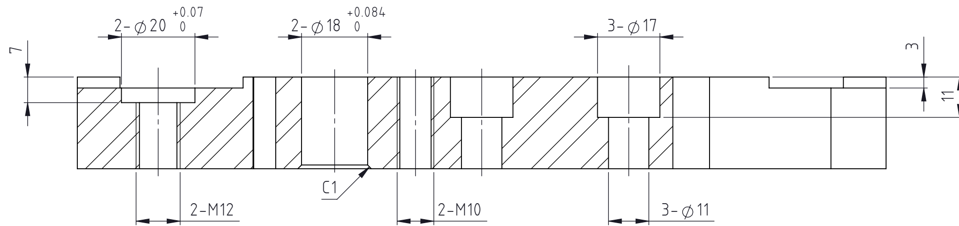
SECTION A-A SCALE 1:1
