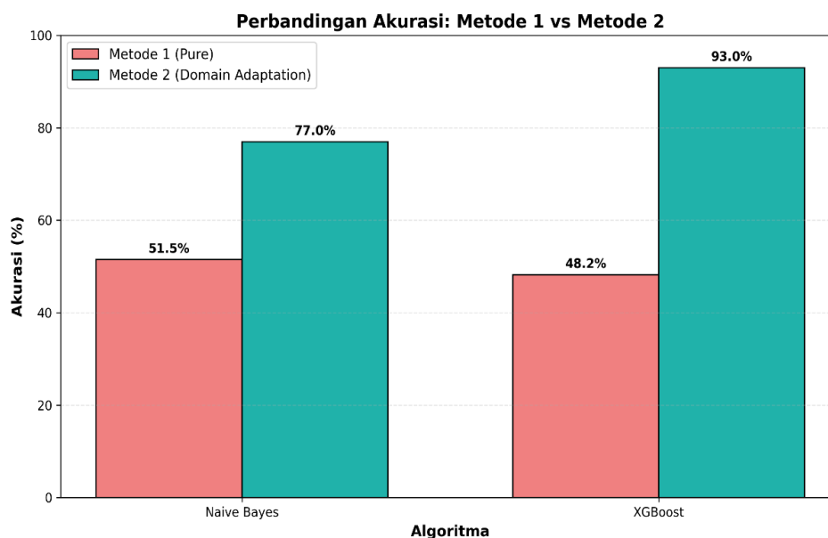
Gambar IV. 9 Perbandingan Akurasi Metode 1 dan Metode 2
