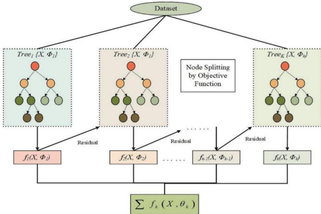
Gambar II. 1 Ilustrasi Additive training pada Arsitektur XGBoost
