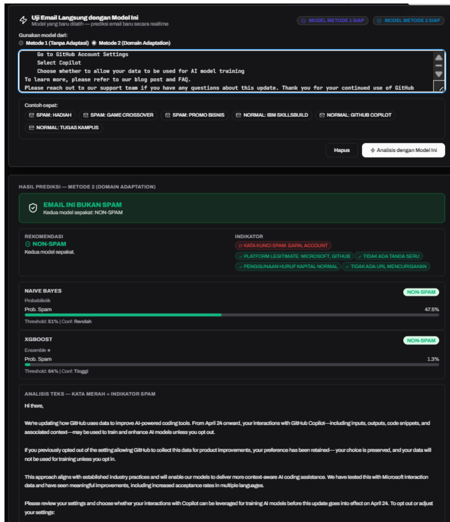
Gambar IV. 21 Tampilan Pengujian Model Hasil Pelatihan
