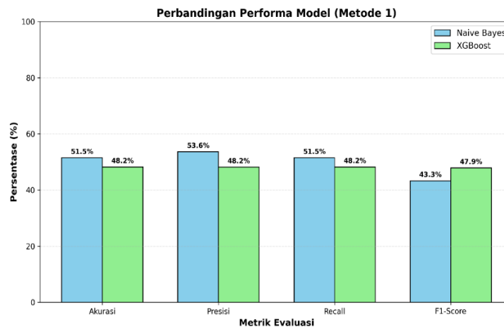
Gambar IV. 5 Perbandingan Metrik Evaluasi Metode 1
