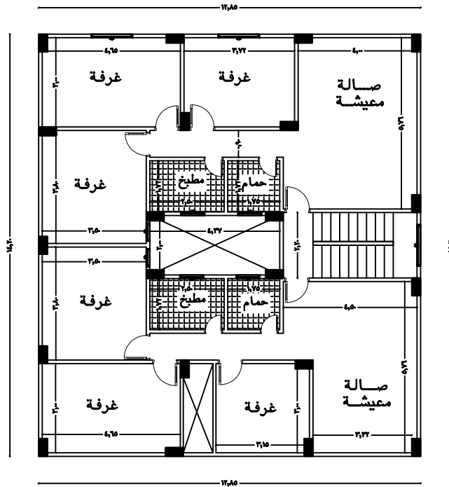
المسقط الأفقي للدور الأرضي للدور أول علوي
