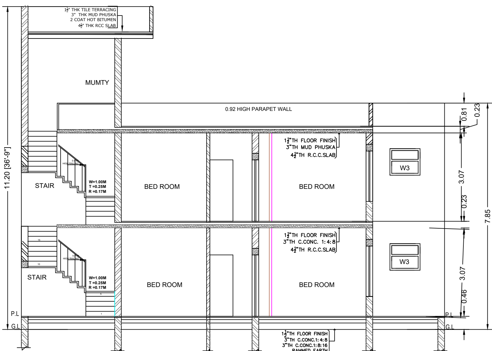
SECTION A-B
