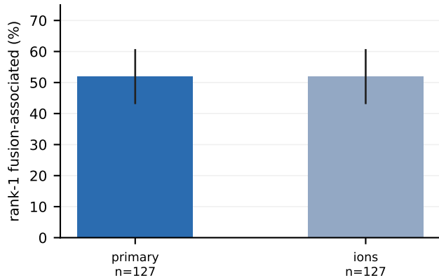
P2Rank
