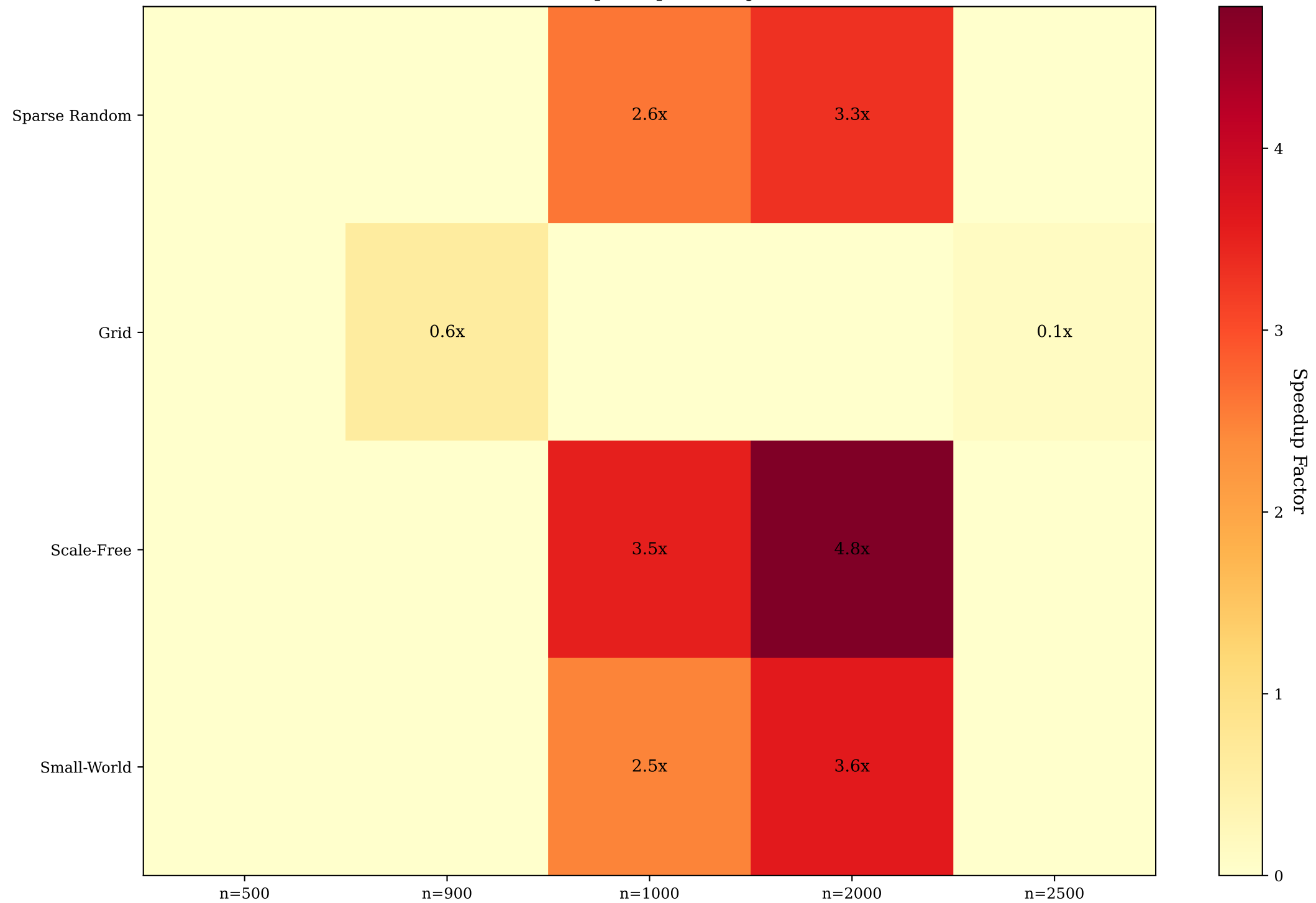
ALSSSP Speedup over Dijkstra
