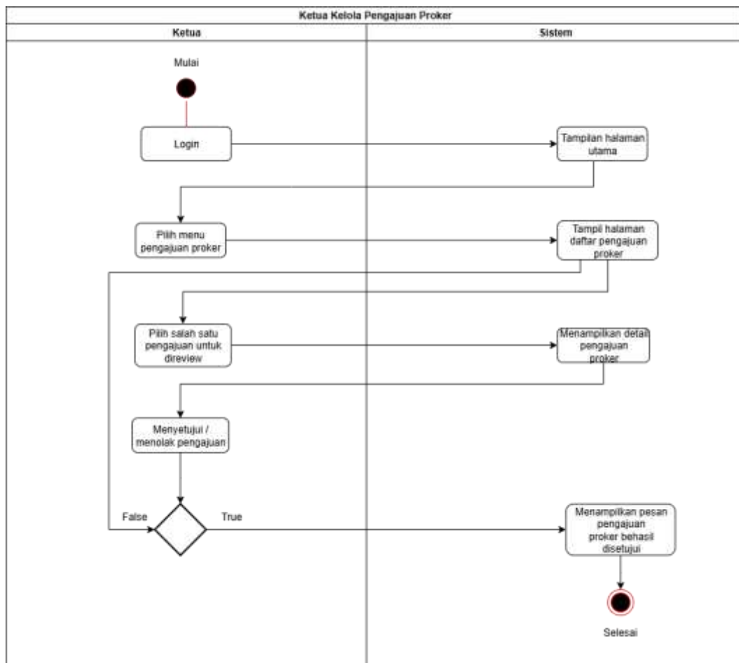
Gambar 4.16 Activity Diagram Ketua Kelola Pengajuan Program Kerja
