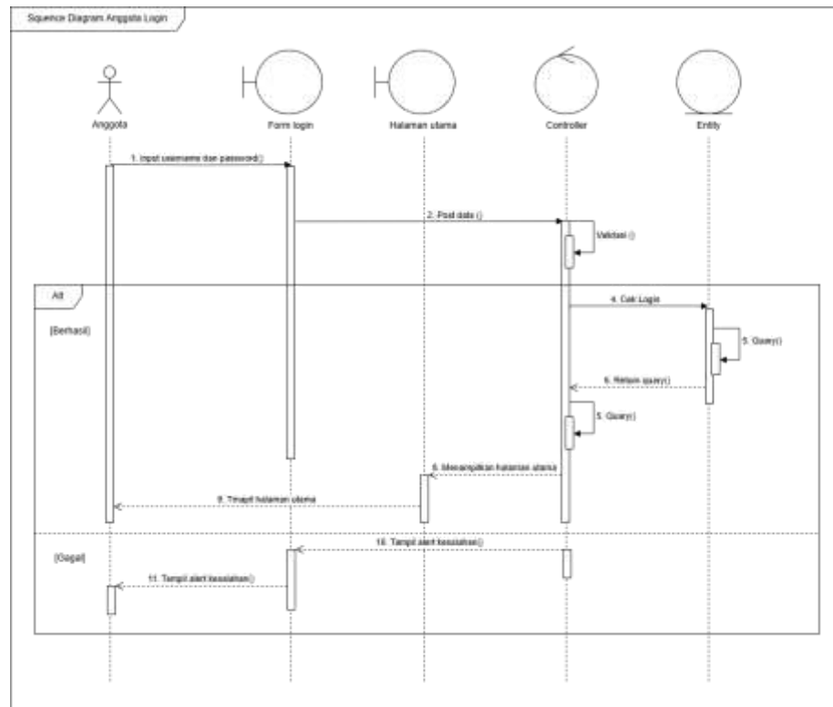
Gambar 4.48 Sequence Diagram Anggota Login
