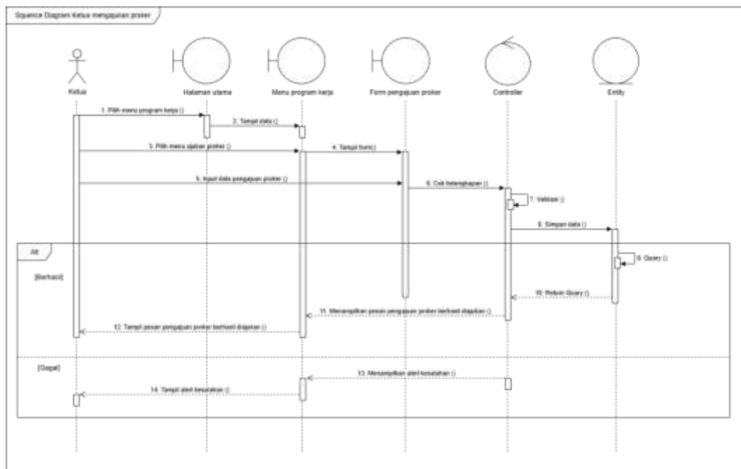
Gambar 4.38 Sequence Diagram Ketua Mengajukan Program Kerja
