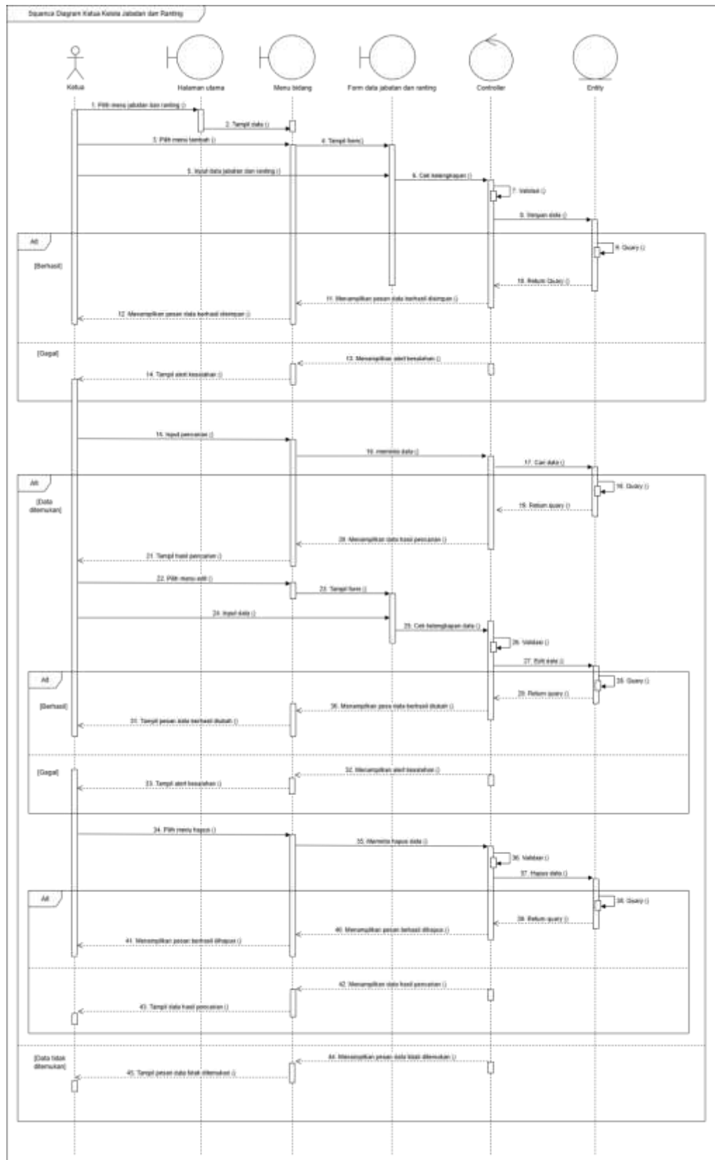
Gambar 4.37 Sequence Diagram Ketua Kelola Jabatan dan Ranting
