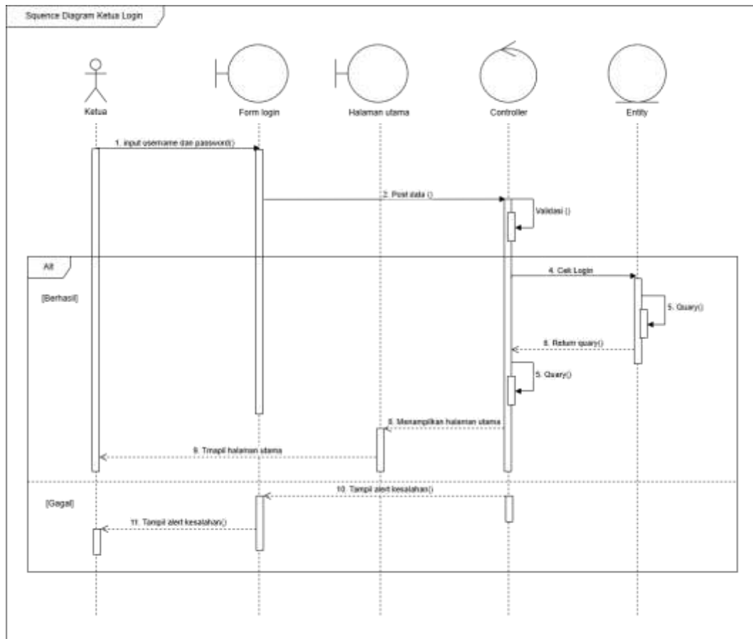
Gambar 4.35 Sequence Diagram Ketua Login
