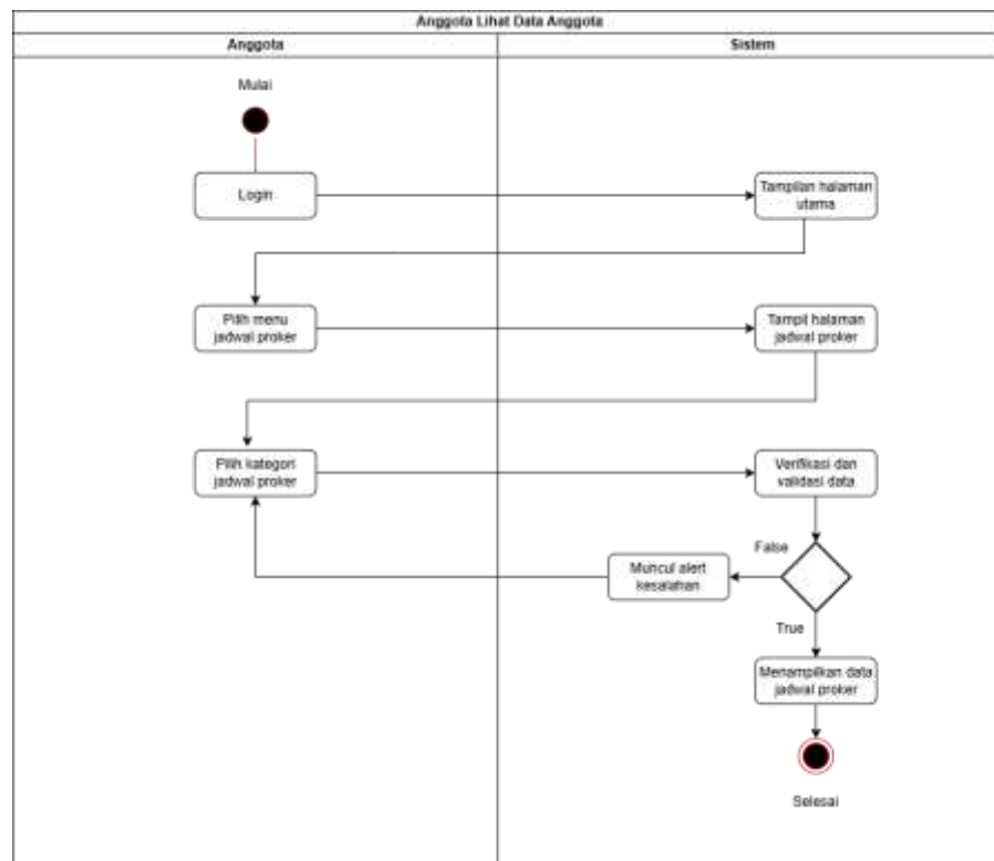
Gambar 4.25 Activity Diagram Anggota Lihat Data Anggota
