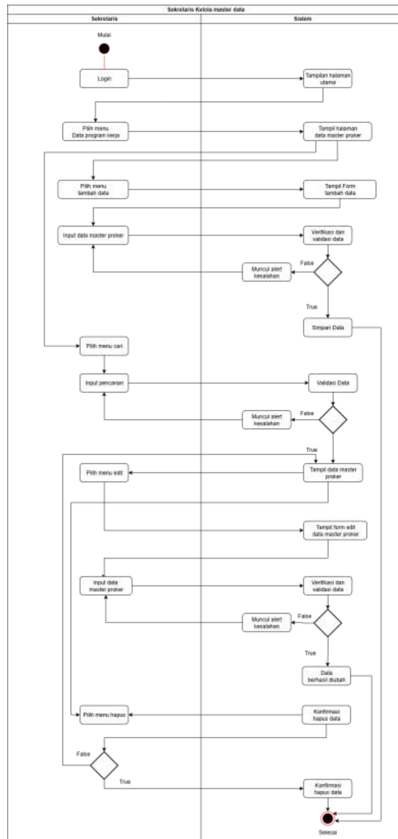
Gambar 4.21 Activity Diagram Sekretaris Kelola Master Data Program Kerja
