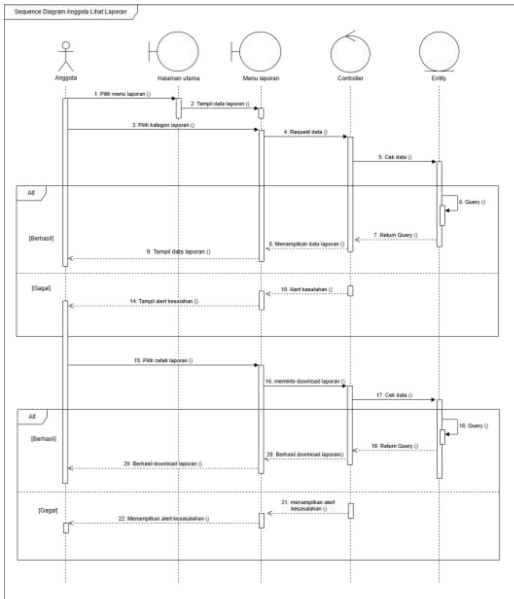
Gambar 4.50 Sequence Diagram Anggota Lihat Laporan
