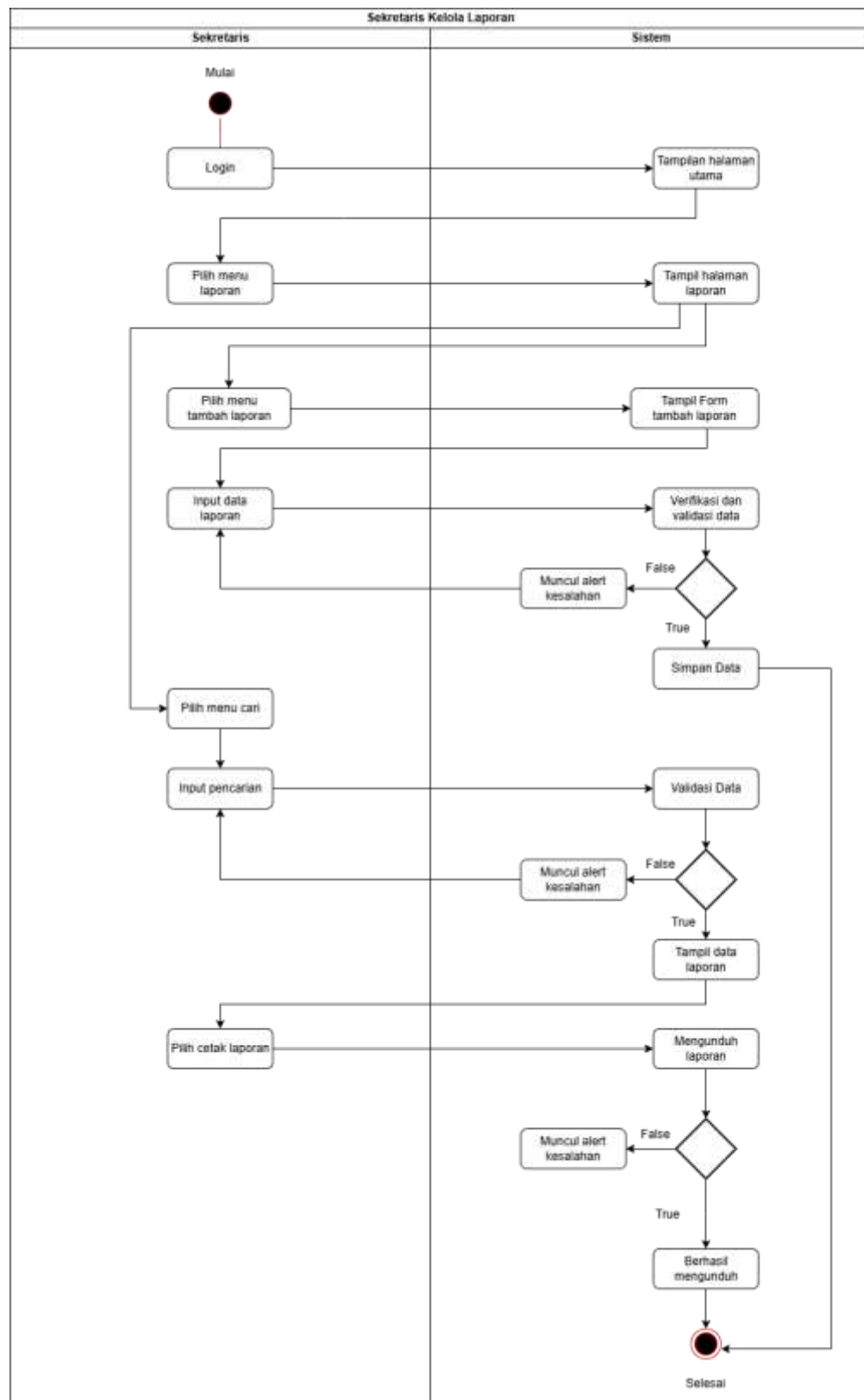
Gambar 4.23 Activity Diagram Sekretaris Kelola Laporan
