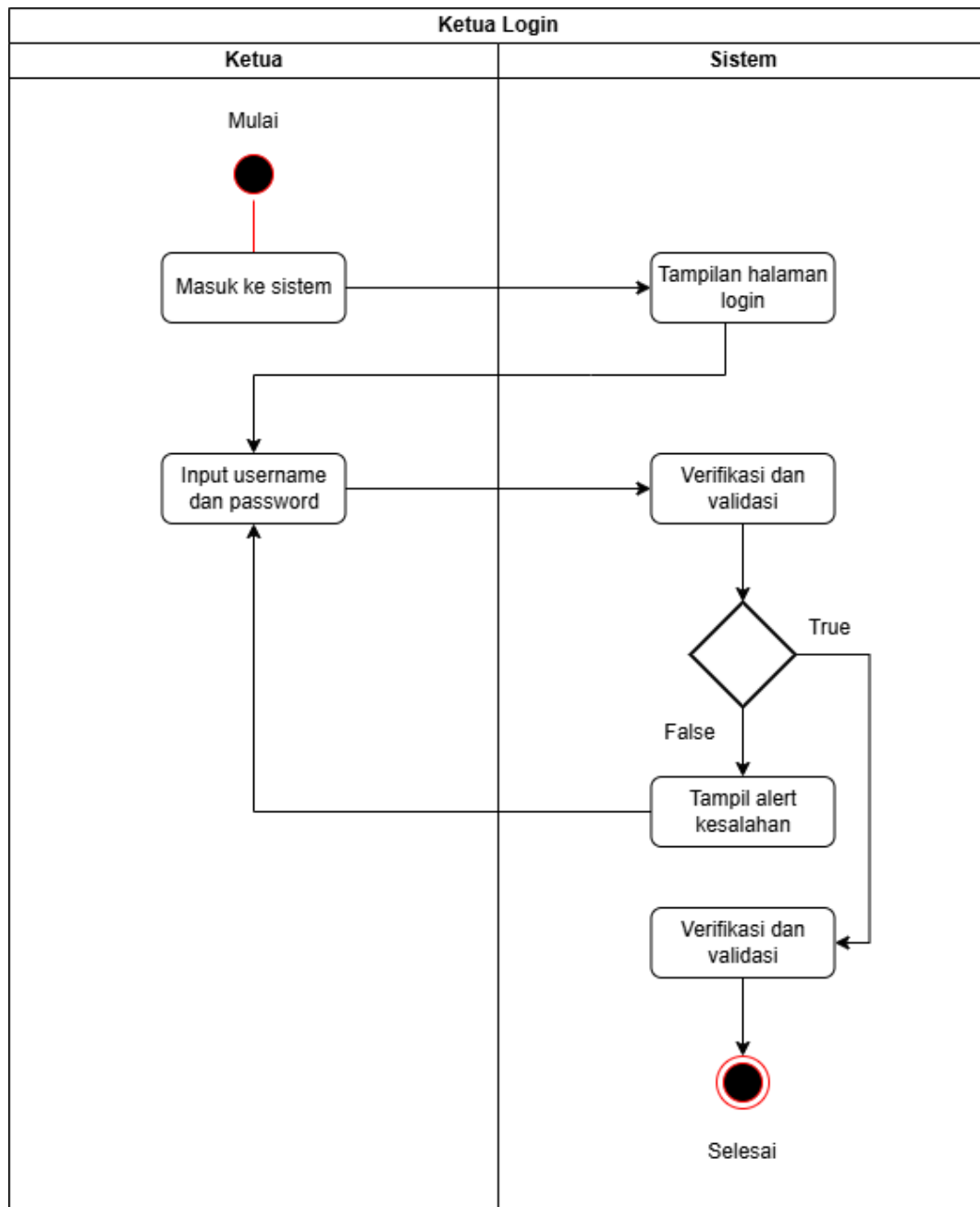
Gambar 4.11 Activity Diagram Ketua Login
