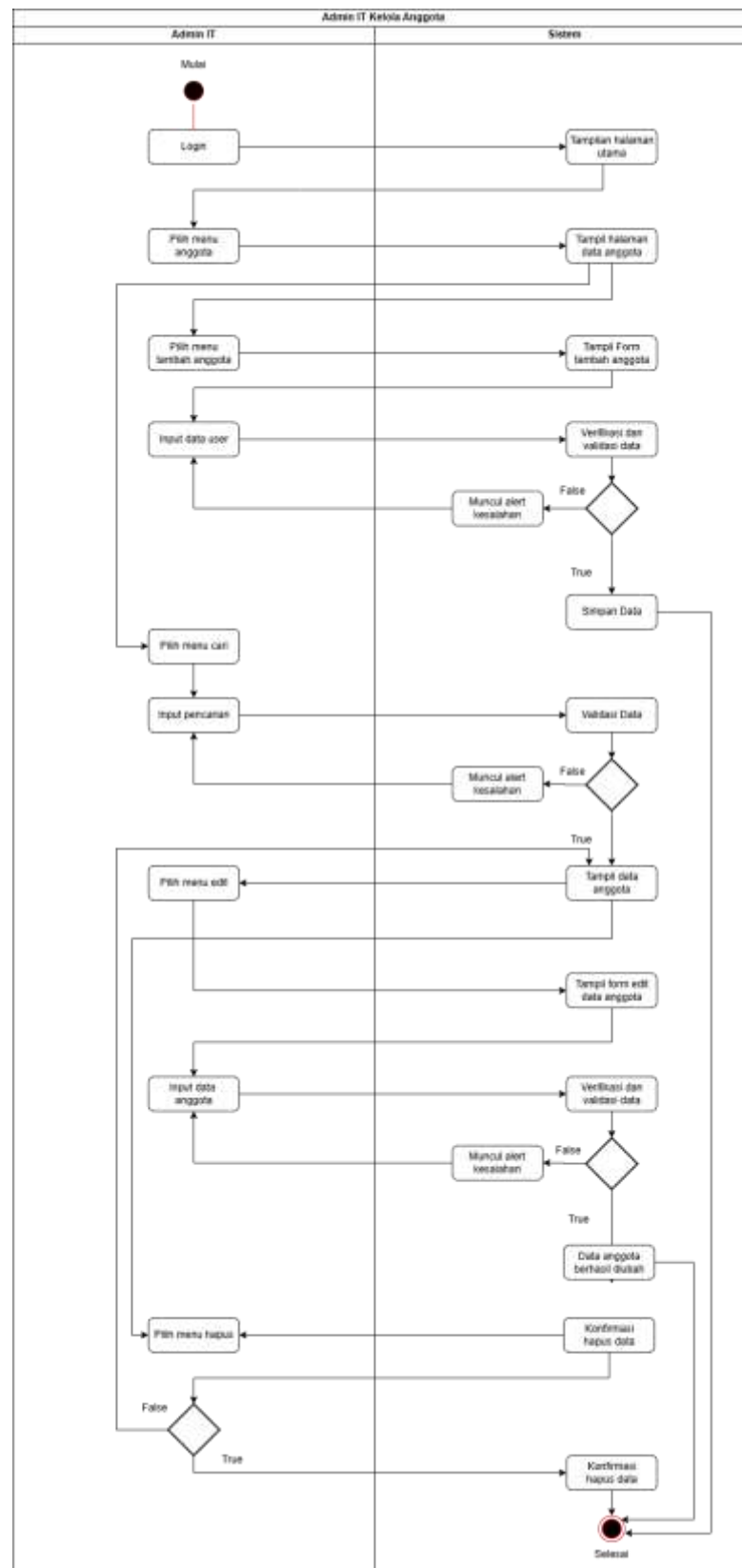
Gambar 4.4 Activity Diagram Admin IT Kelola User dan Anggota
