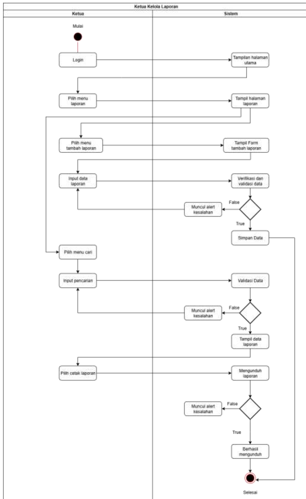
Gambar 4.18 Activity Diagram Ketua Kelola Laporan
