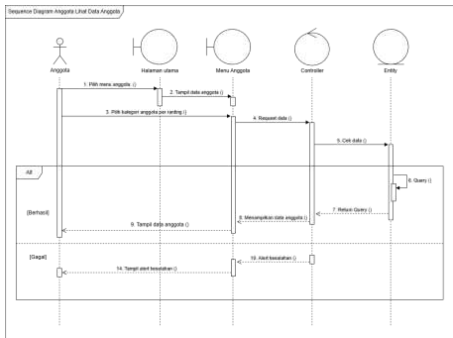
Gambar 4.49 Sequence Diagram Anggota Lihat Data Anggota
