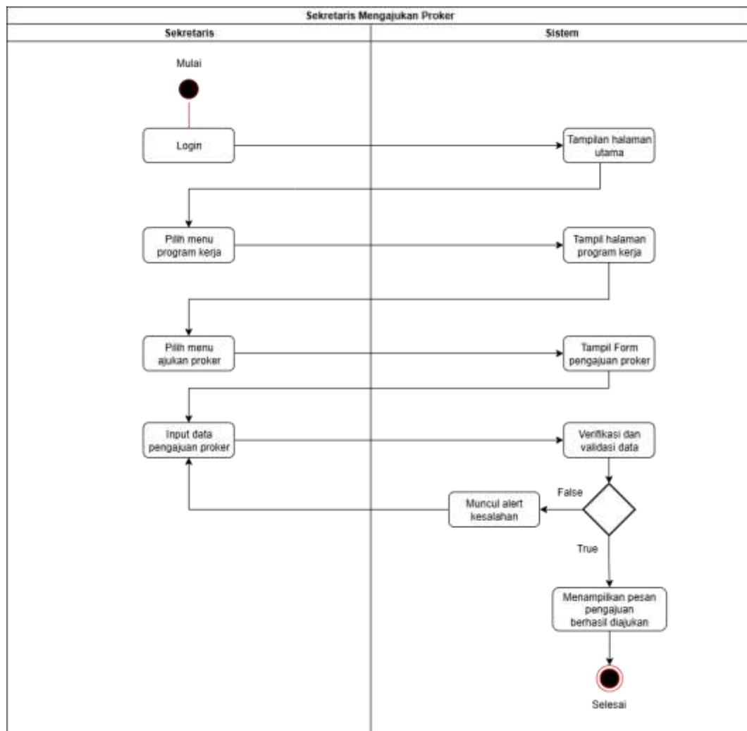
Gambar 4.22 Activity Diagram Sekretaris Mengajukan Proker
