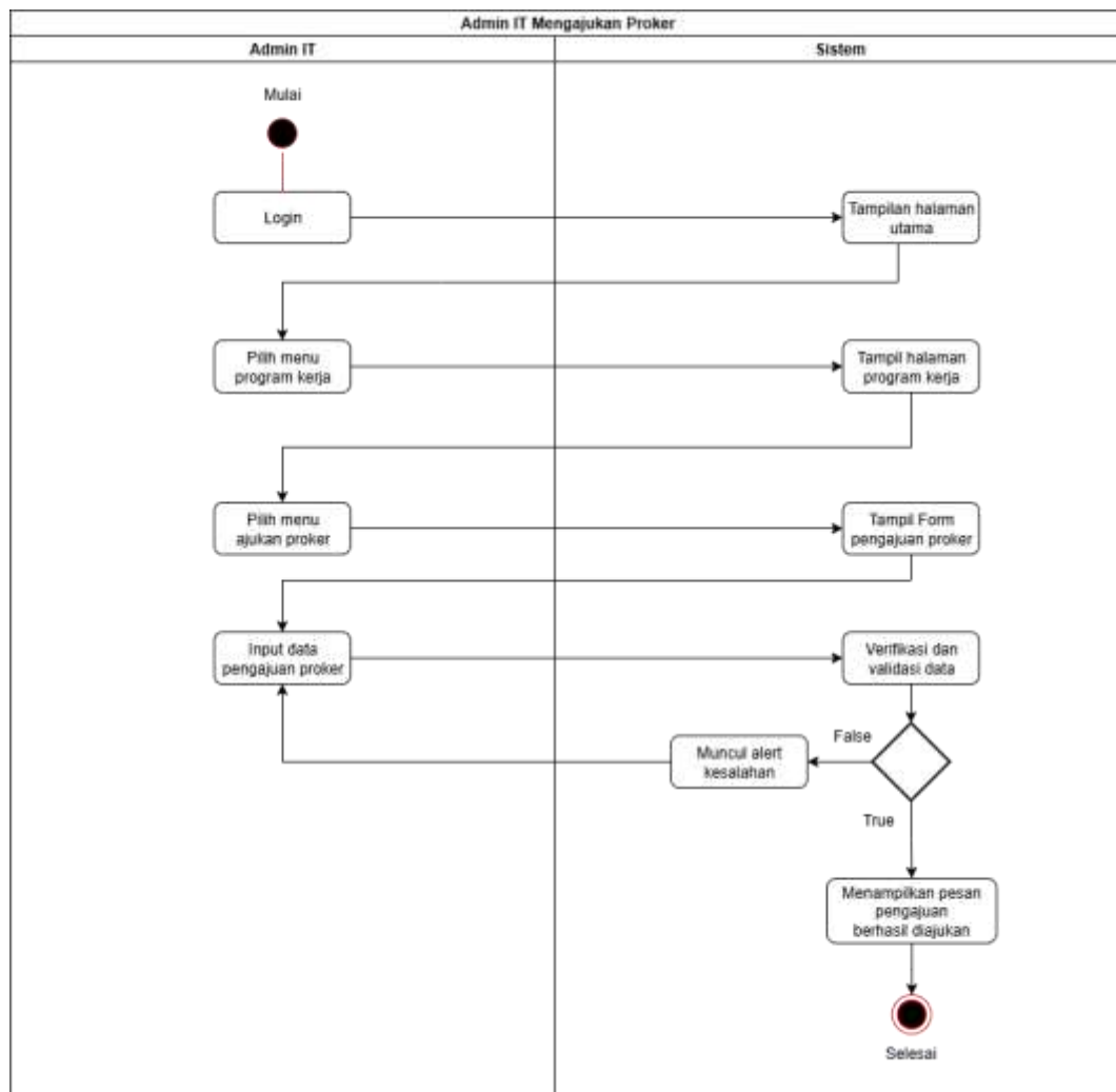
Gambar 4.6 Activity Diagram Admin IT Mengajukan Program Kerja
