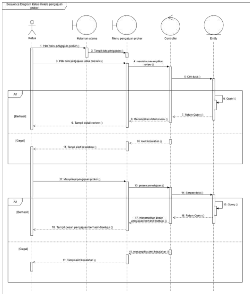
Gambar 4.40 Sequence Diagram Ketua Kelola Pengajuan Program Kerja
