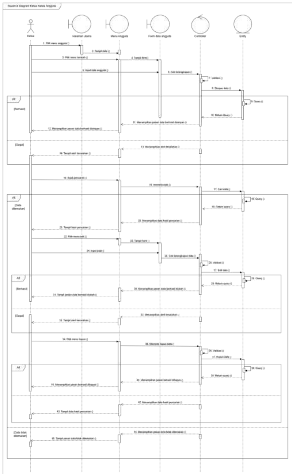
Gambar 4.36 Sequence Diagram Ketua Kelola User dan Anggota
