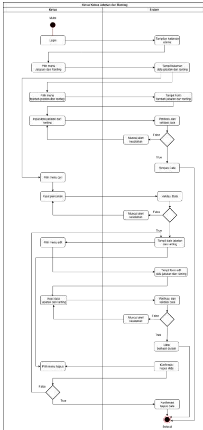
Gambar 4.13 Activity Diagram Ketua Kelola Jabatan dan Ranting
