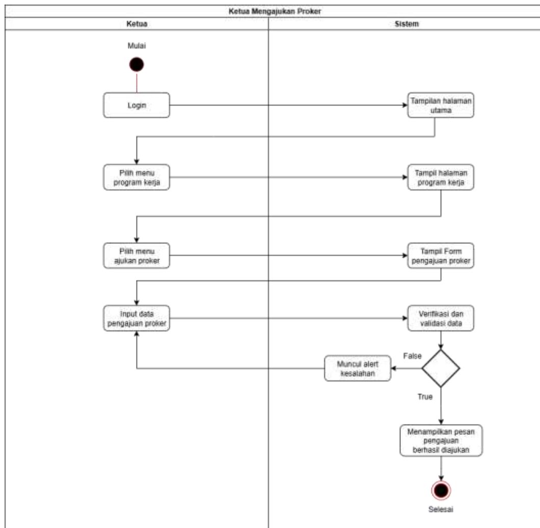
Gambar 4.14 Activity Diagram Ketua Mengajukan Program Kerja
