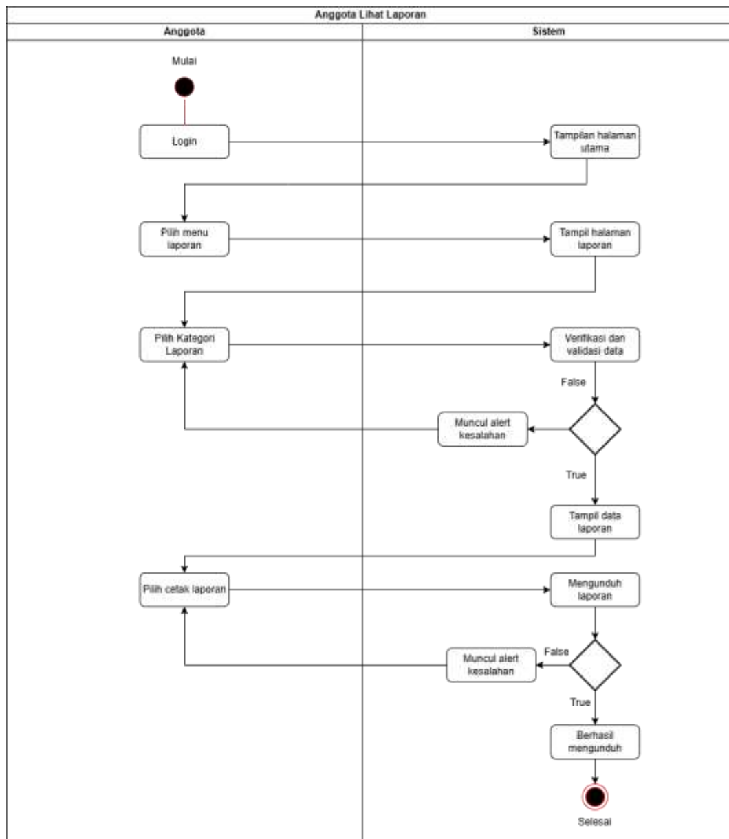
Gambar 4.26 Activity Diagram Anggota Lihat Laporan
