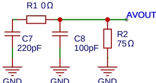
AV OUT
