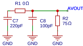
AV OUT
