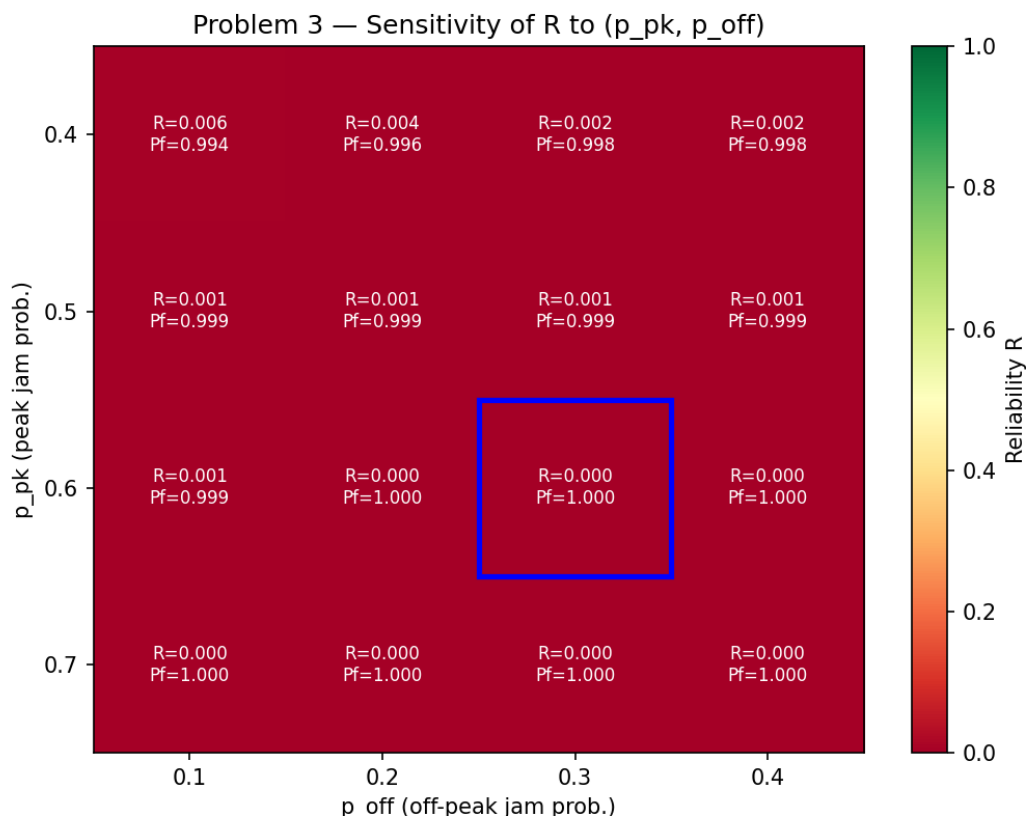
图 7.4 敏感性扫描热力图
