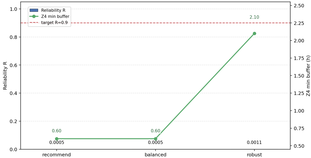
图 7.1 三方案 R/P_{\text{fail}} 对比
