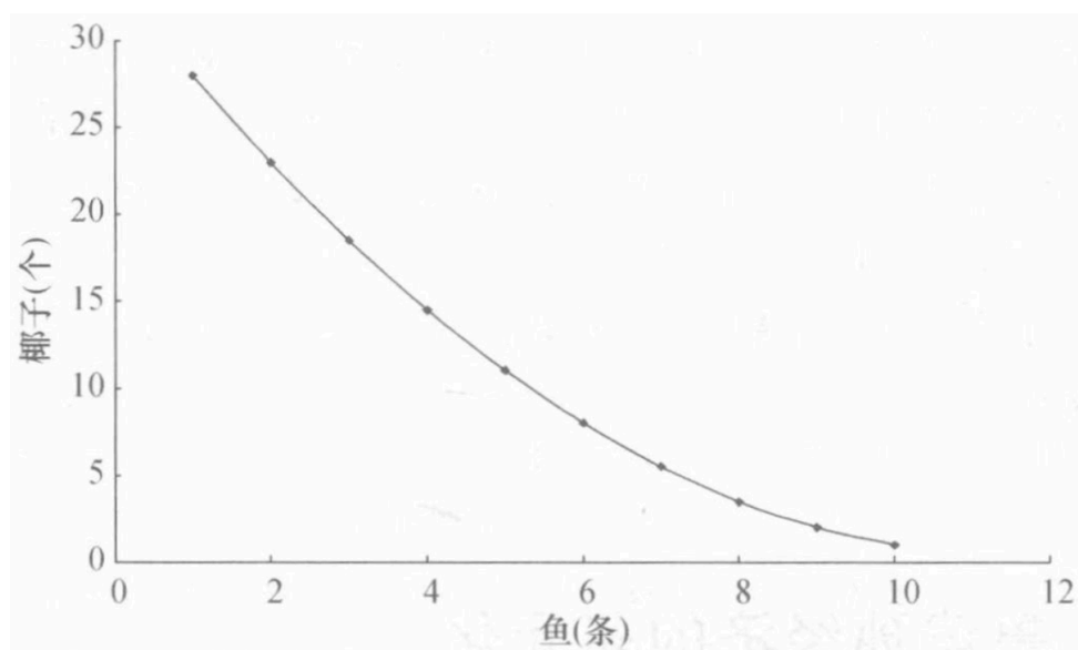
图 2.5: 无差异曲线
