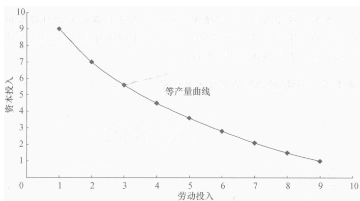
图 5.7: 等产量曲线
