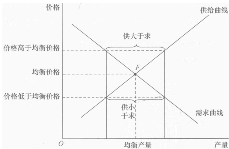
图 6.3: 非均衡状态
