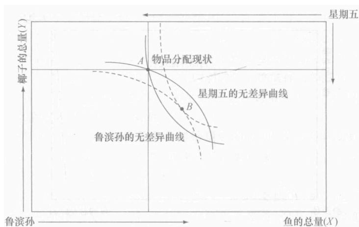
图 3.2: 交换的机理
