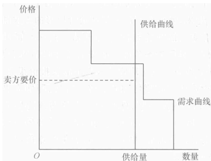
图 6.8: 一口价
