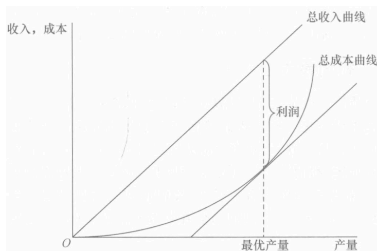
图 5.1: 利润最大化
