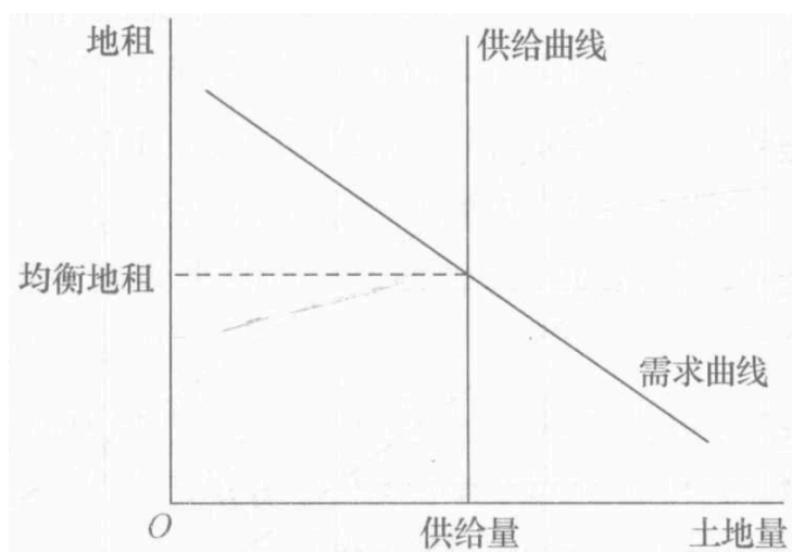
图 7.26: 地租的决定
