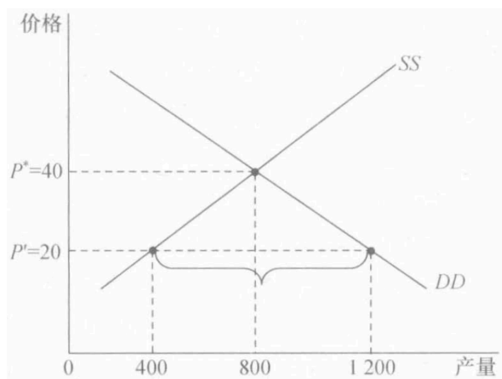
图 6.12: 最高限价
