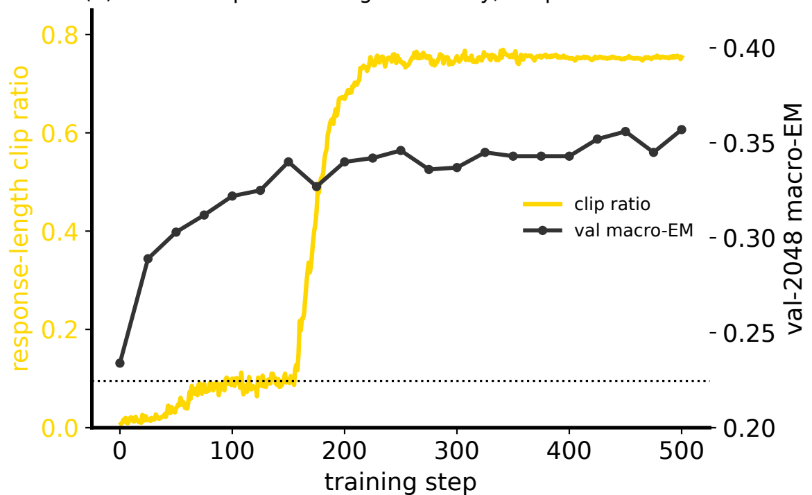
(b) HCAPO: clip \rightarrow 0.75 length runaway, EM plateaus \approx 0.35
