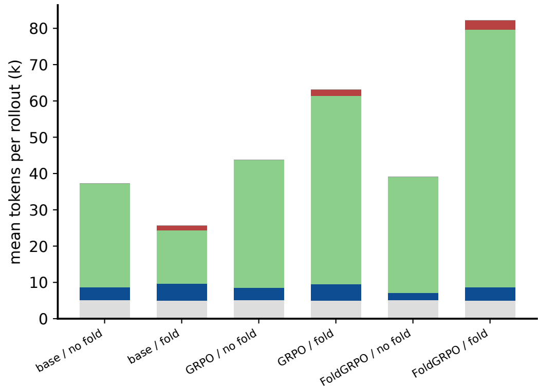
t1n4
