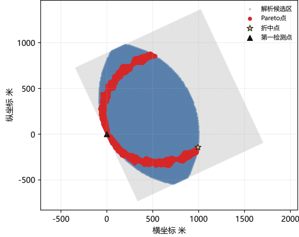
图 2 第二检测点条件保证候选区、Pareto 点与参考站址（程序图中的“解析候选区”“折中点”分别对应本文的条件保证区与参考站址）
