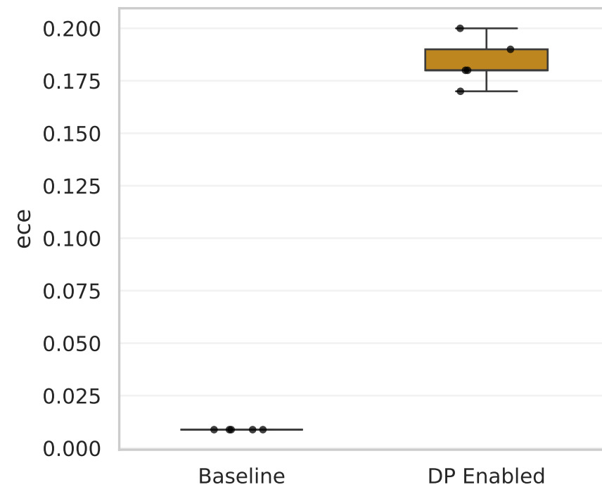
ECE
