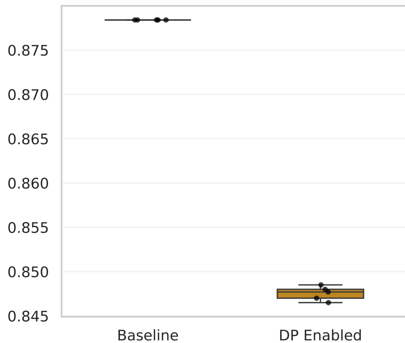
AUROC
