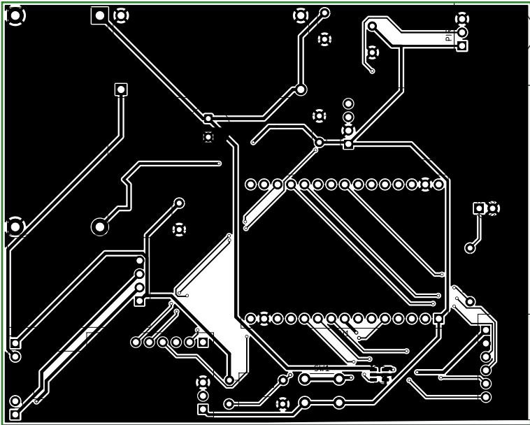
TOP LAYER (Components & F.Silks)
