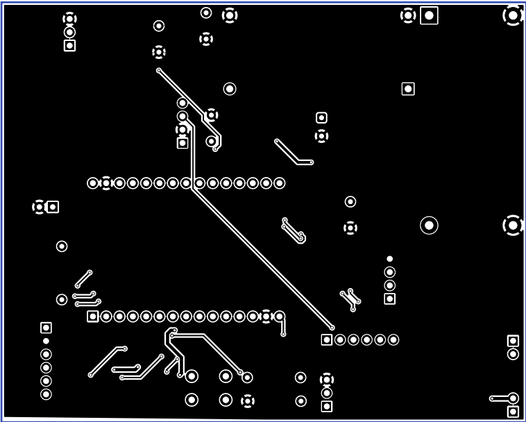
BOTTOM LAYER (Traces & B.Cu Plane)
