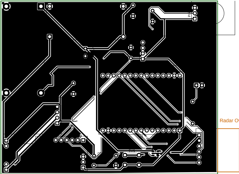
TOP LAYER (Components & F.Silks)
