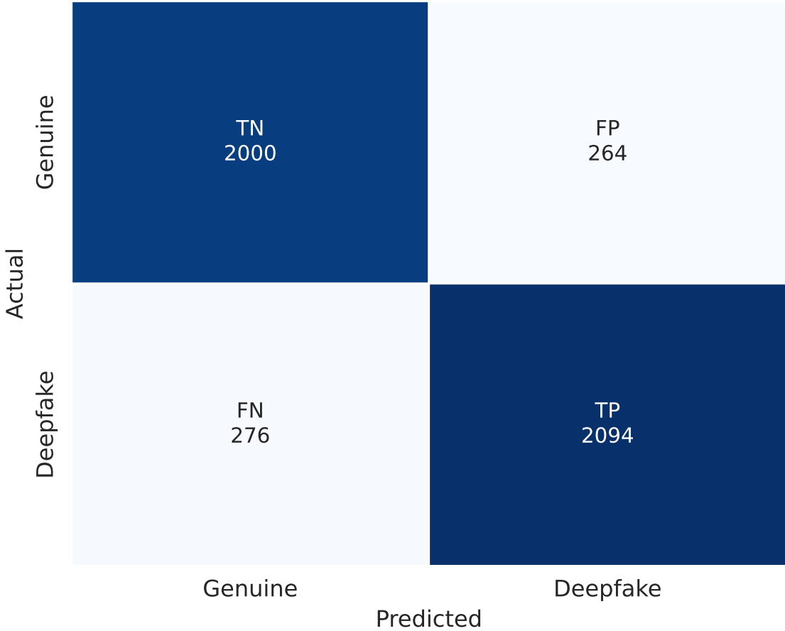
ResNet34 + MelSpec Acc=88.3% | EER=11.7% | F1=88.6%
