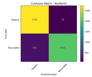
(d) Confusion Matrix
