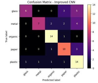
(d) Confusion Matrix
