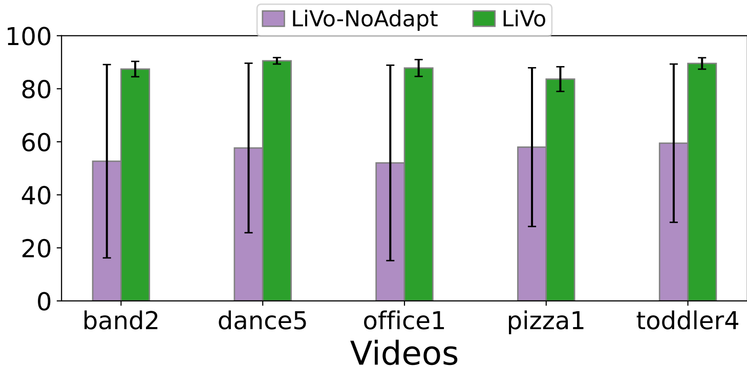
PSSIM Geometric
