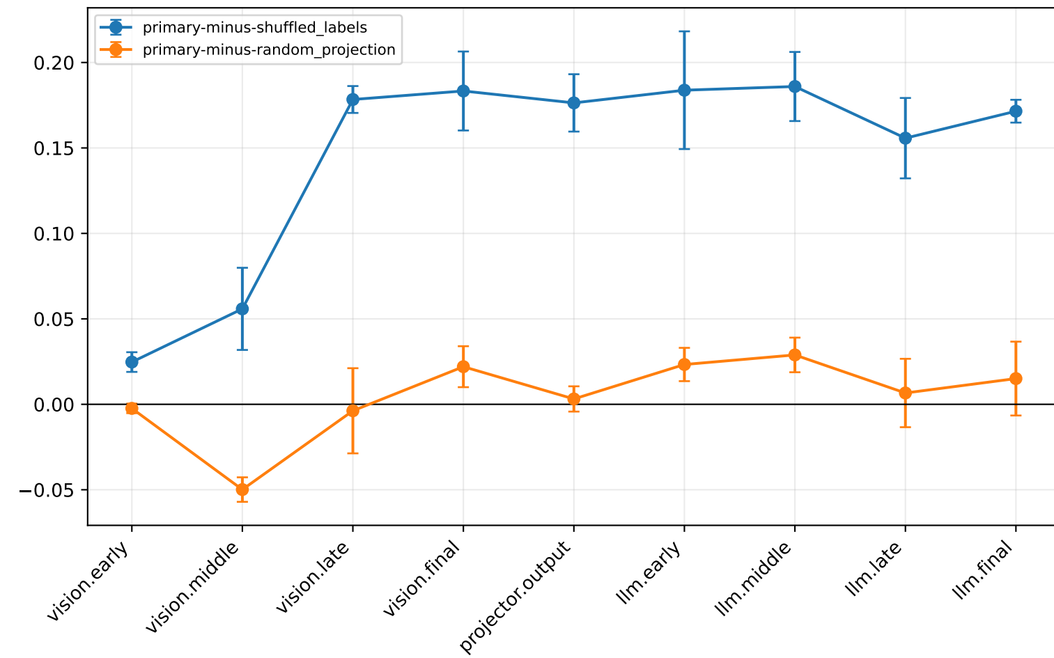
Paired F1 differences: mean \pm seed SD
